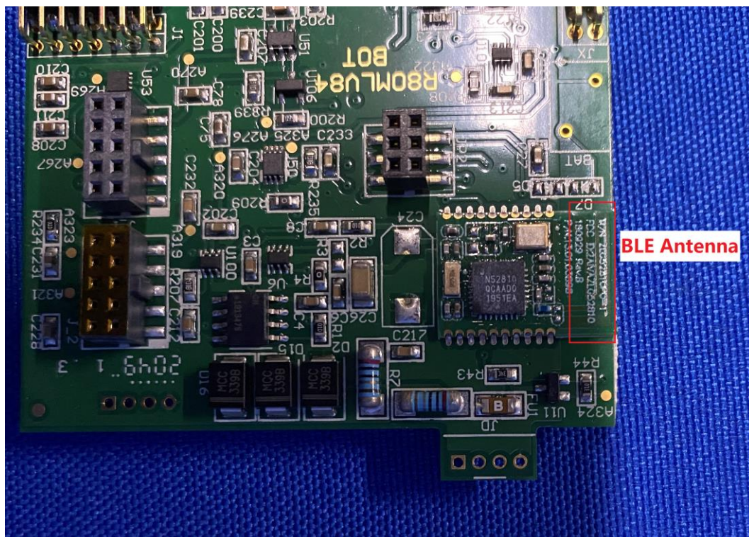
(6) EUT Photo
