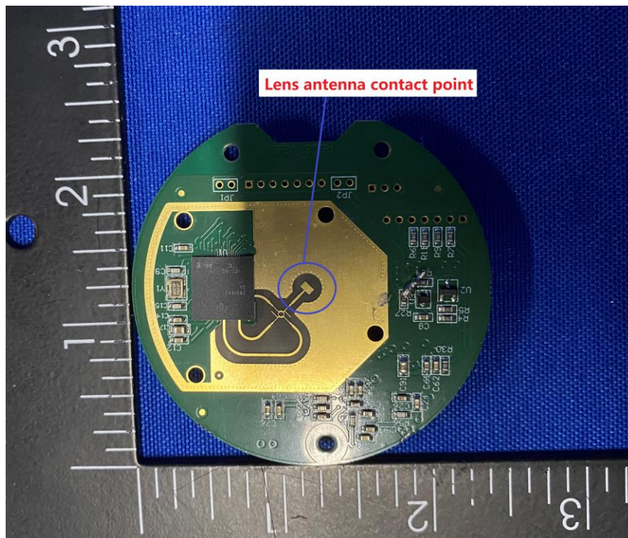
(14) EUT Photo
