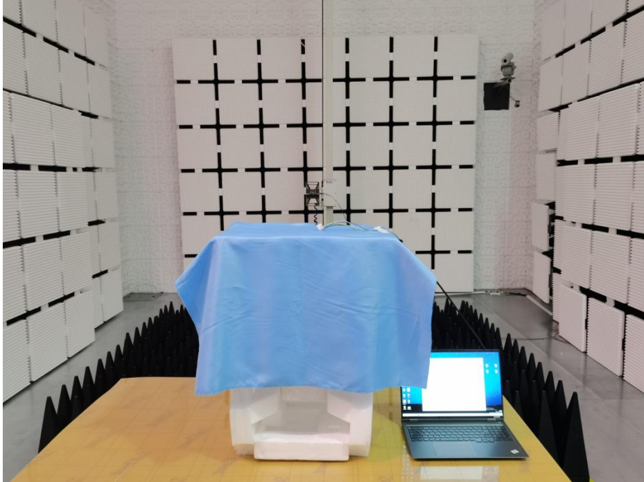
RSE Test Photo (1GHz-18GHz)
