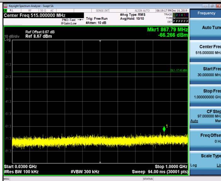
BLE_BT4.0_Ant1_2402_30~1000
