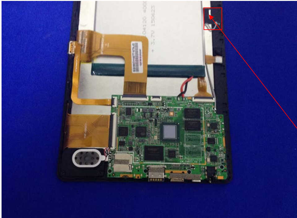
WIFI&BT Antenna
