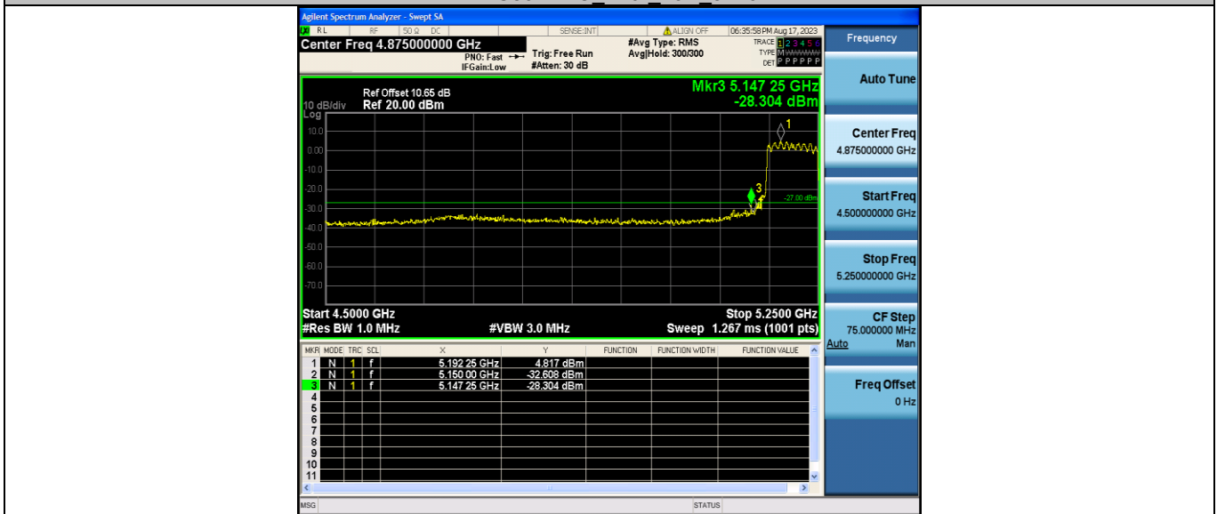
11AC80MIMO_Ant2_Low_5210
