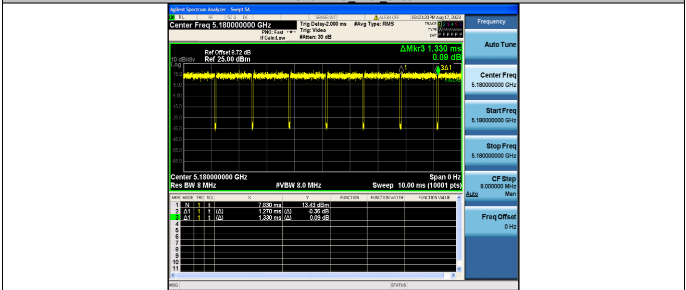
11AC20MIMO_Ant2_5180
