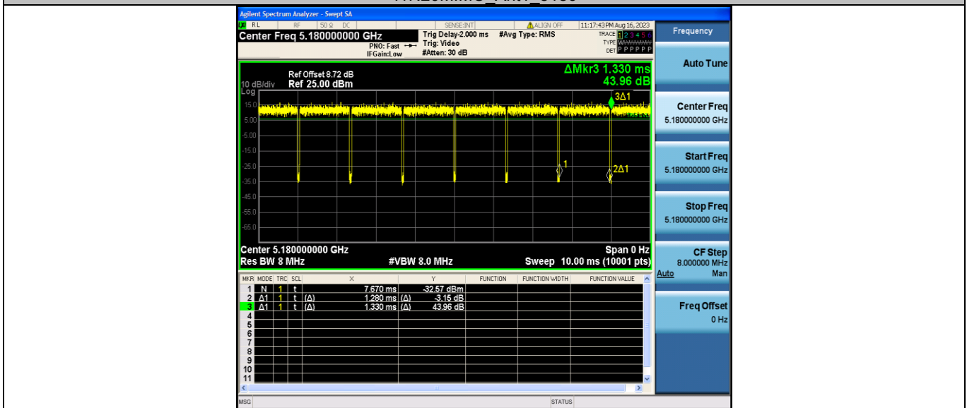
11N20MIMO_Ant2_5180
