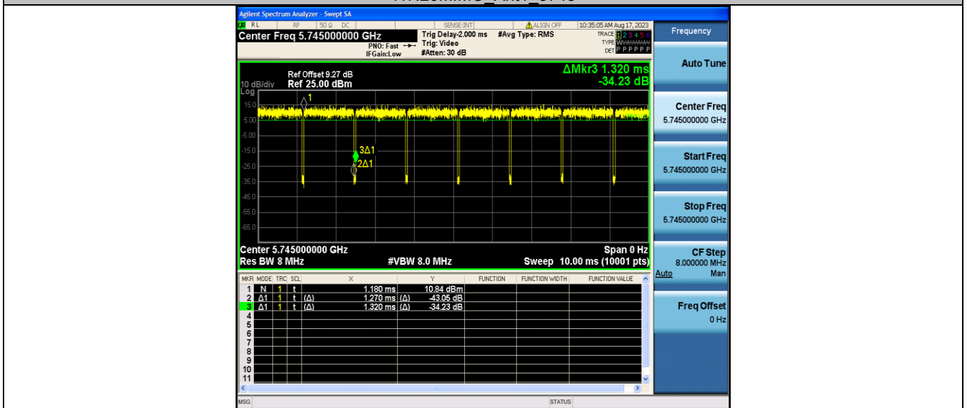
11N20MIMO Ant2 5745
