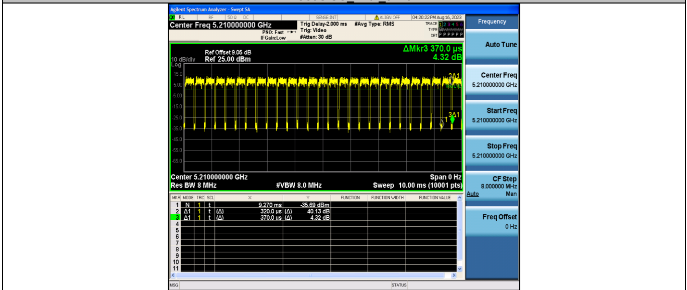
11AC80SISO_Ant2_5210
