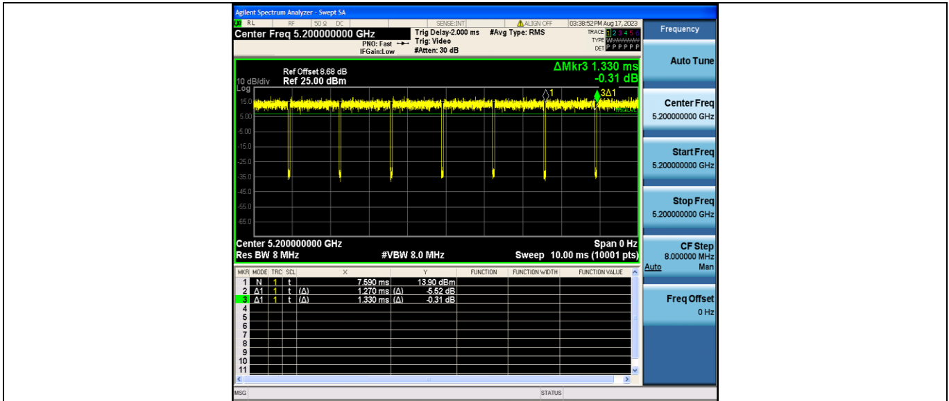
11AC20MIMO_Ant2_5200
