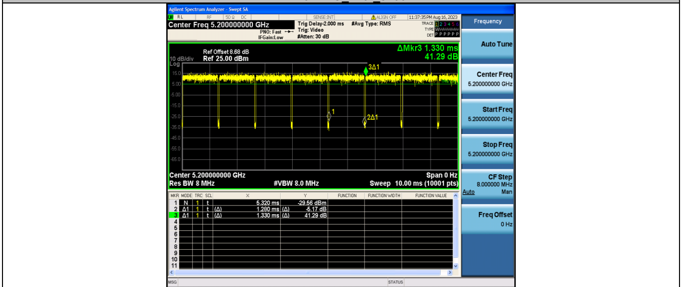
11N20MIMO Ant2 5200
