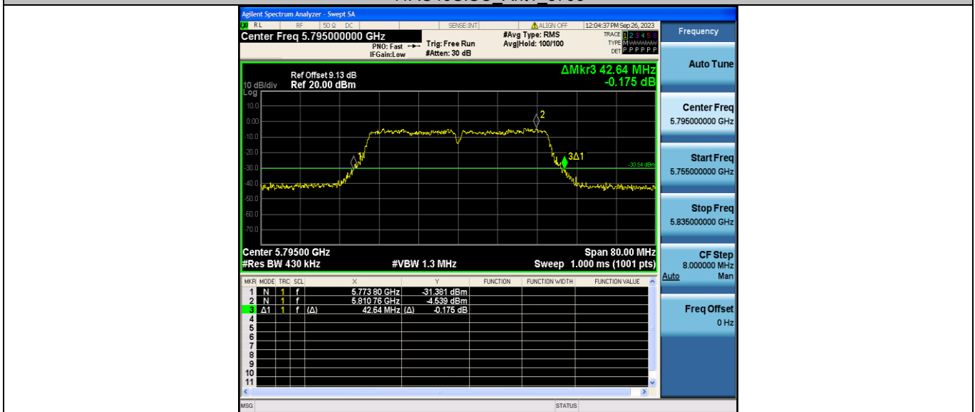
11AC40SISO_Ant2_5795
