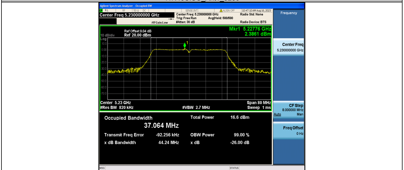
11N40SISO_Ant2_5230
