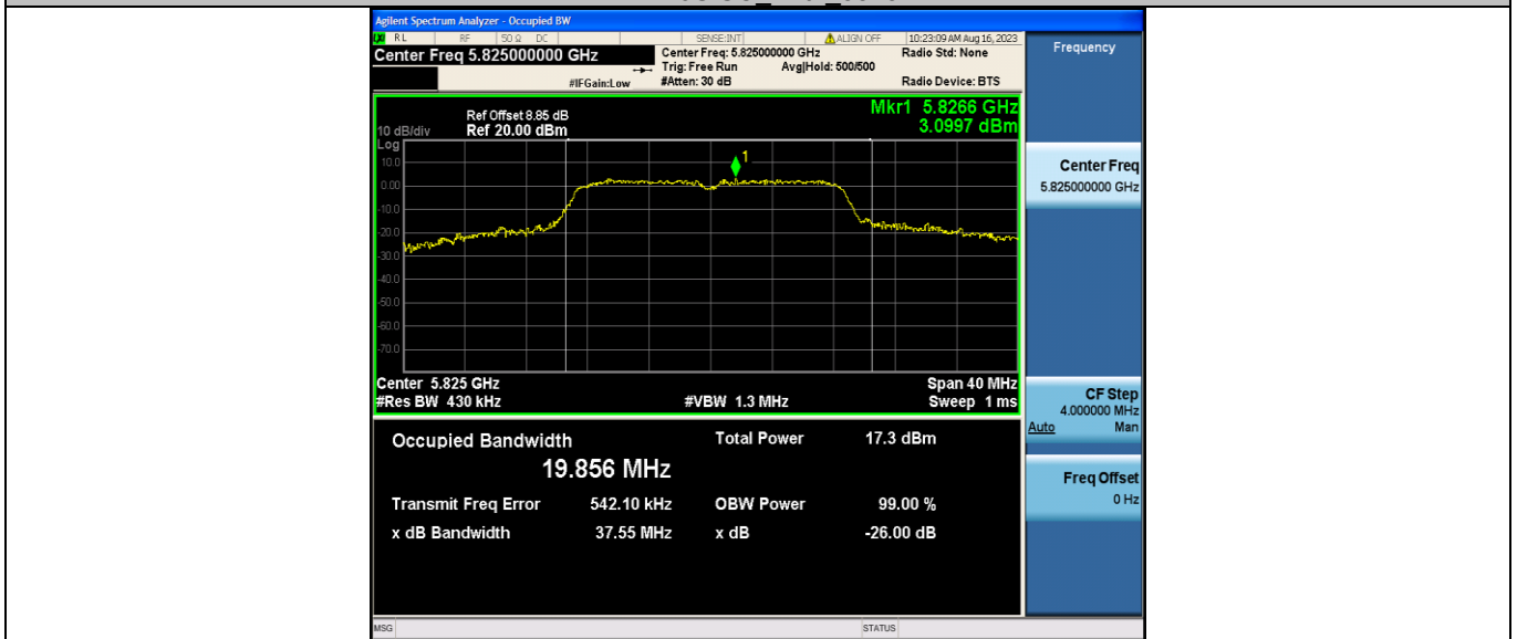
11N20SISO_Ant2_5825
