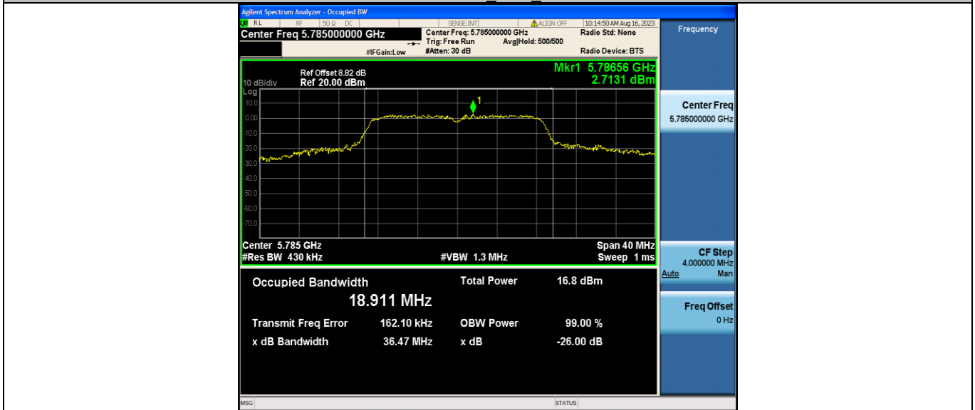
11N20SISO_Ant2_5785
