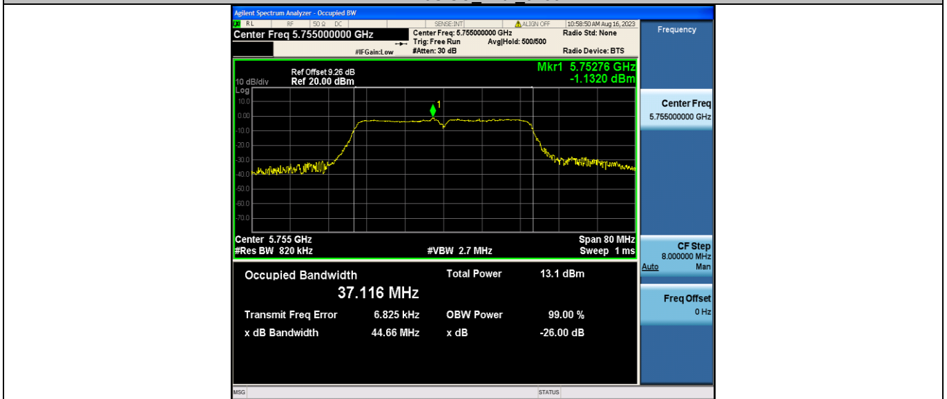
11N40SISO_Ant2_5755
