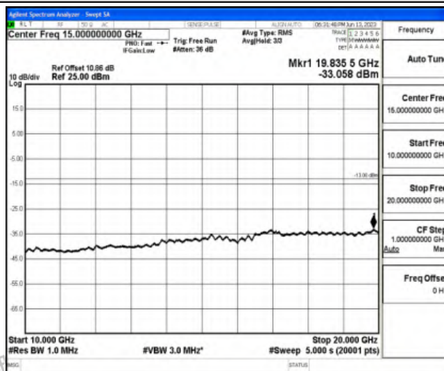
Band25-3MHz-QPSK-26365-1RB#0-Range5:10000~20000MHz
