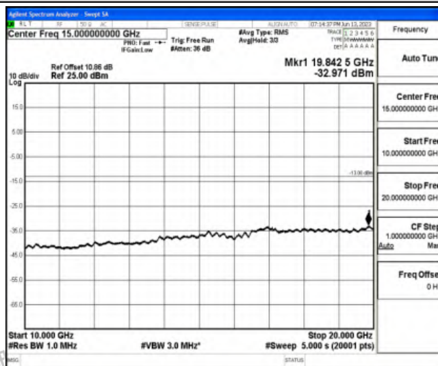
Band25-20MHz-QPSK-26590-1RB#0-Range5:10000~20000MHz
