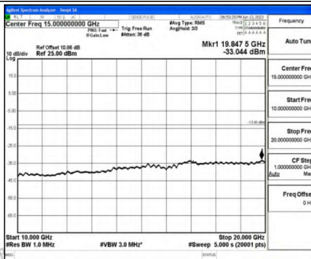
Band25-10MHz-16QAM-26365-1RB#0-Range5:10000~20000MHz
