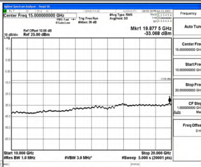
Band25-10MHz-QPSK-26365-1RB#0-Range5:10000~20000MHz
