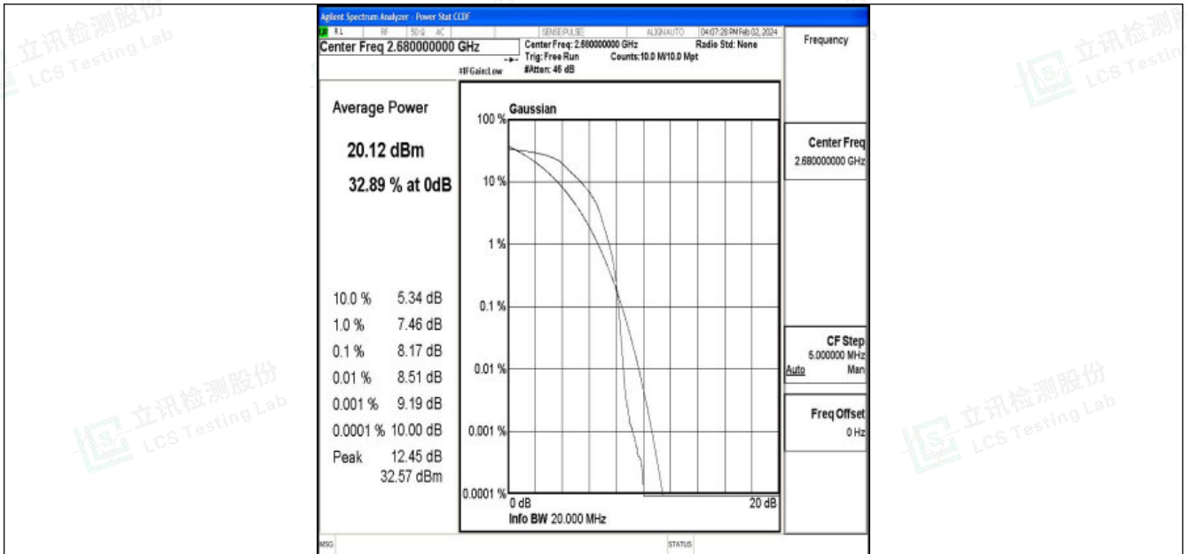
Band41-20MHz-QPSK-41490-1RB#0-PASS
