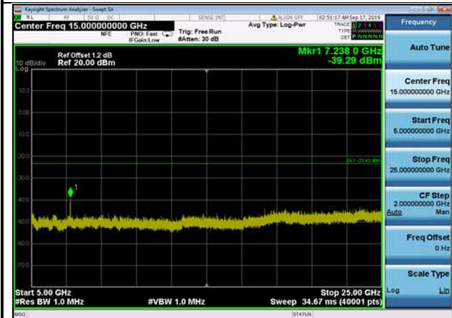
802.11b,2412MHz,Ant0,Plot 5,5000MHz~25000MHz
