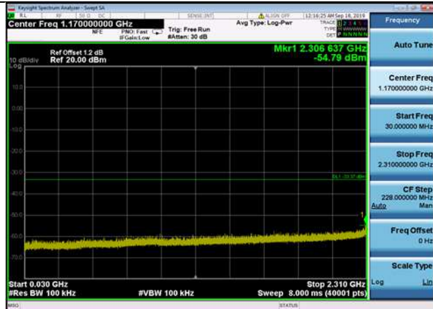
802.11n(HT40),2437MHz,Ant0,Plot 3,30MHz~2310MHz
