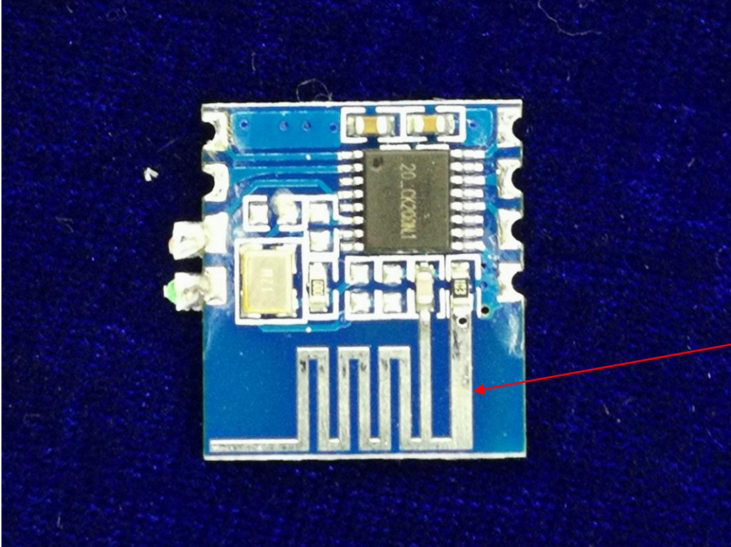
Antenna
