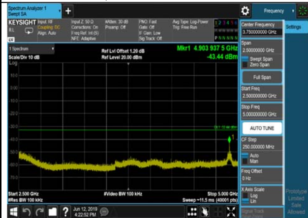
802.11n(HT40),2452MHz,Ant1,Plot 4,2500MHz~5000MHz
