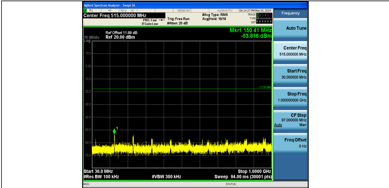
BLE_2M-Ant1-2402-30~1000-PASS
