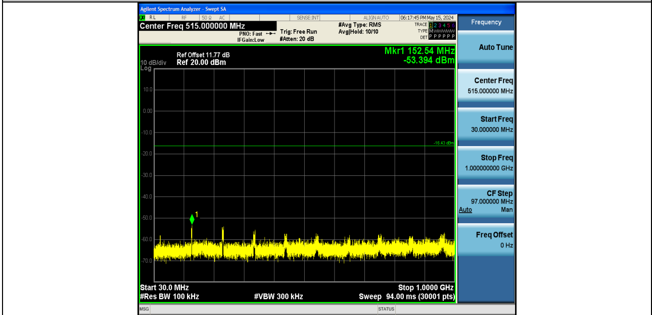
BLE_2M-Ant1-2440-30~1000-PASS
