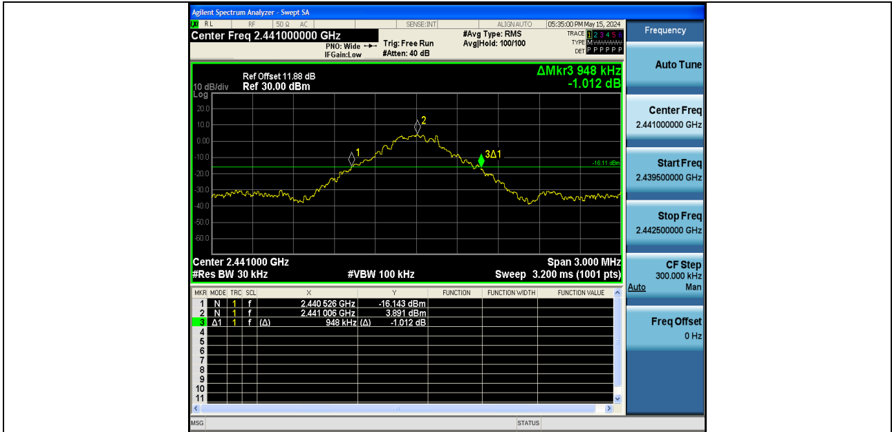
DH5-Ant1-2441
