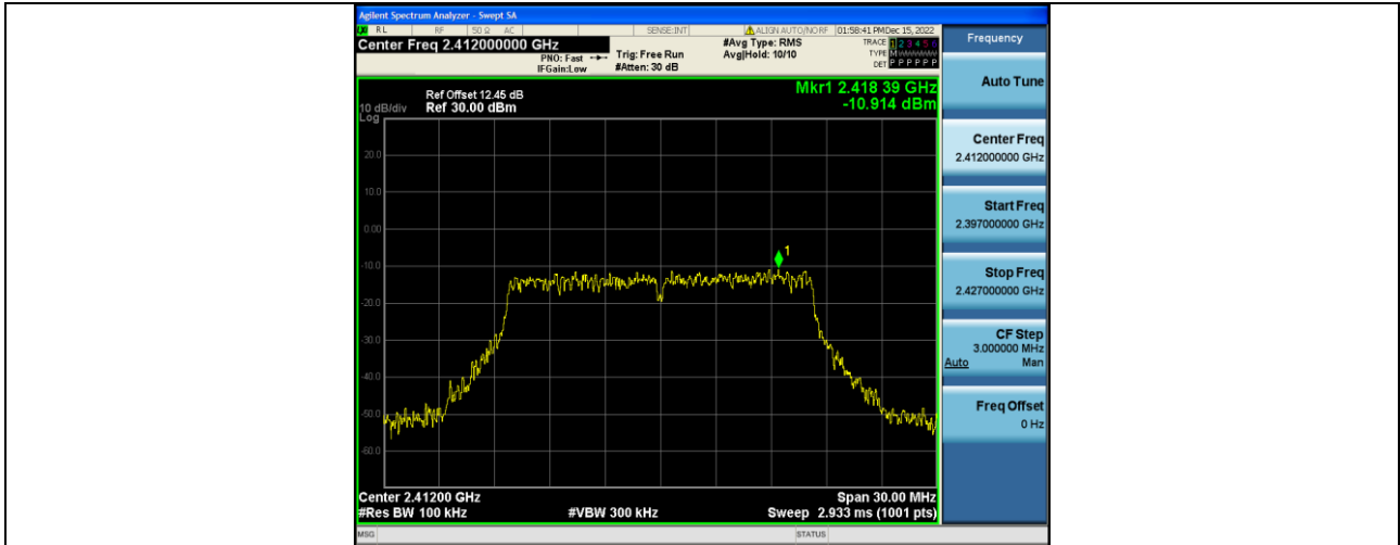
11G-Ant1-2412-30~1000--10.91
