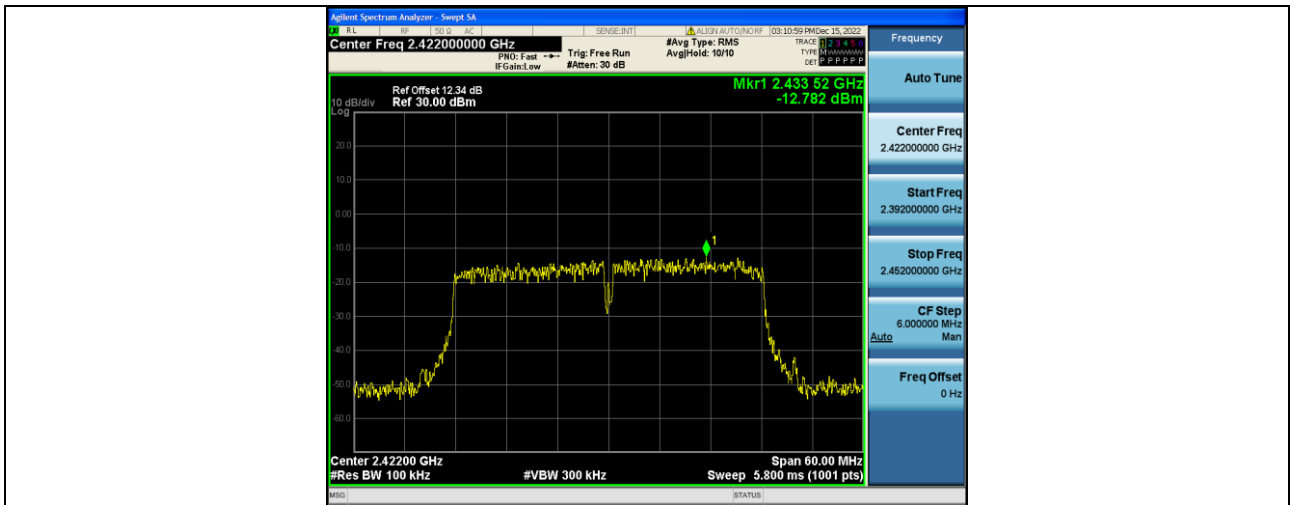
11N40SISO-Ant1-2422-30~1000--12.78
