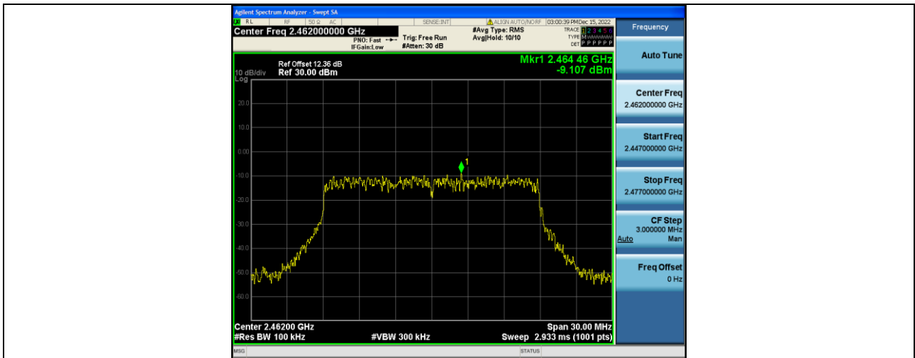
11N20SISO-Ant1-2462-30~1000--9.11
