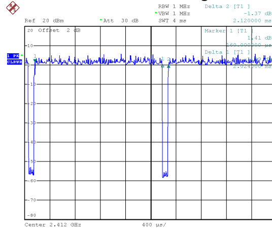
IEEE 802.11g
