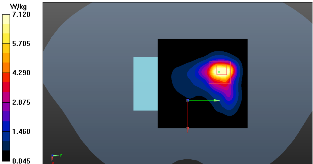
Fig.37 WCDMA Band 2 Body
