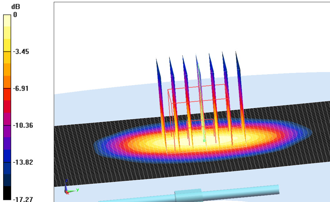
Fig.I.5-2 validation 2600MHz 250mW
