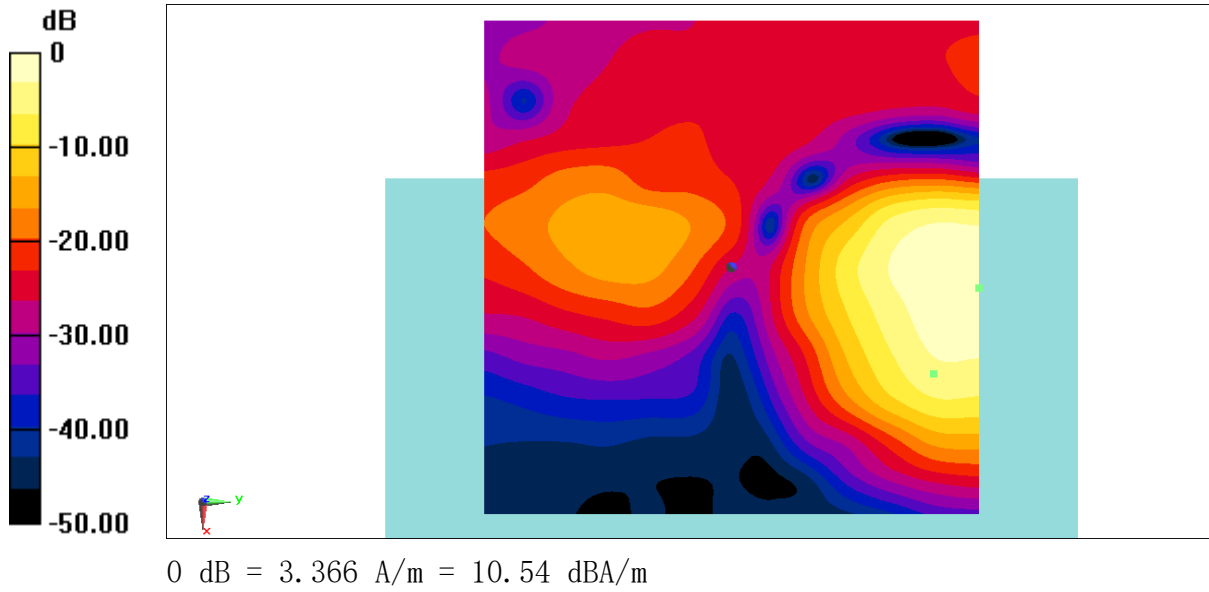
Fig B.10 T-Coil EDGE 850
