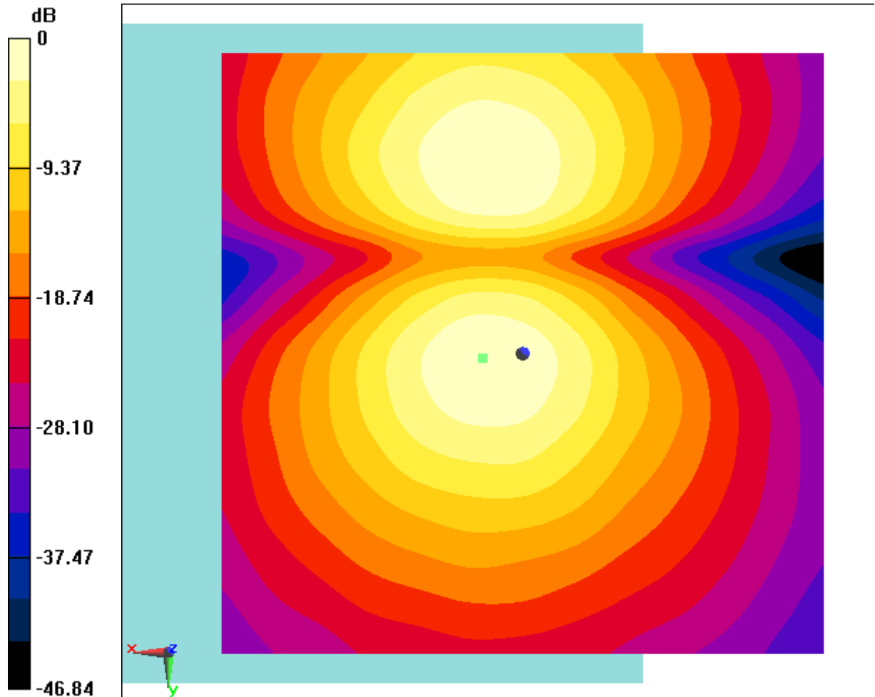
Fig B.15 T-Coil LTE B5
