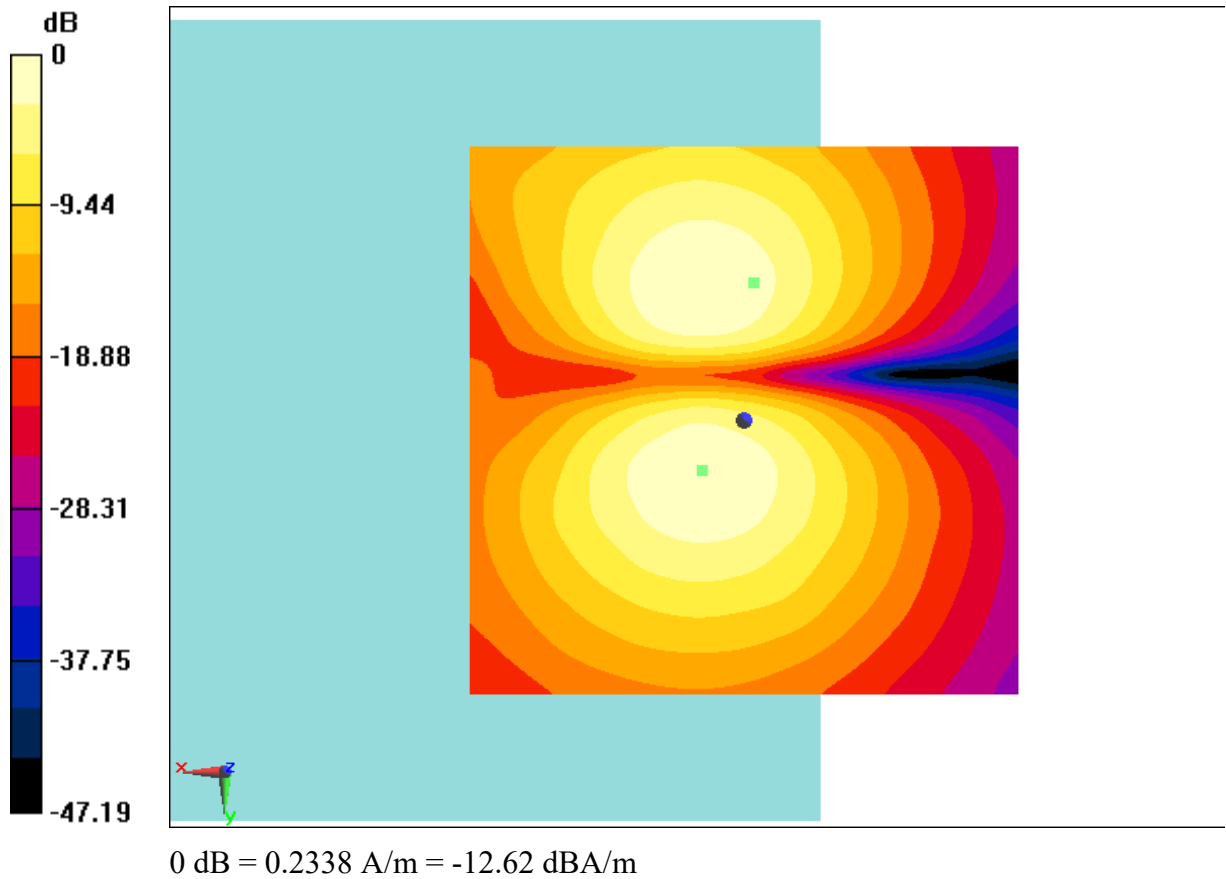
Fig B.25 T-Coil WiFi-2. 4G
