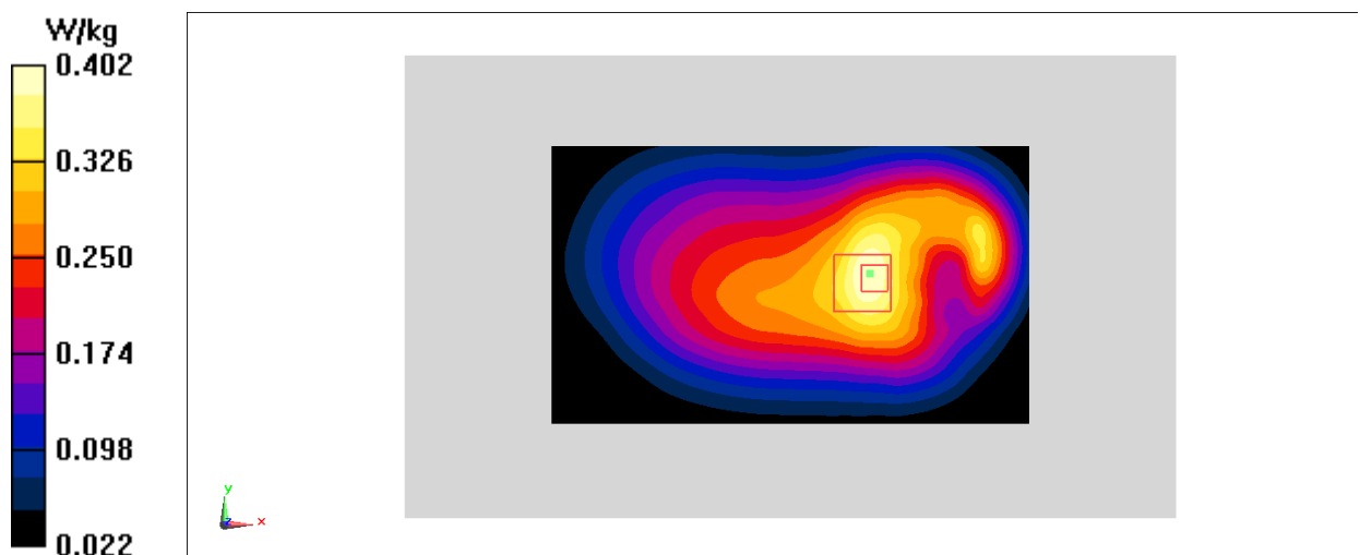
Fig.30 LTE Band26
