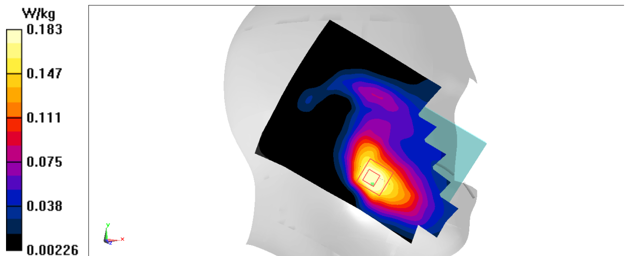
Fig.26 LTE Band4
