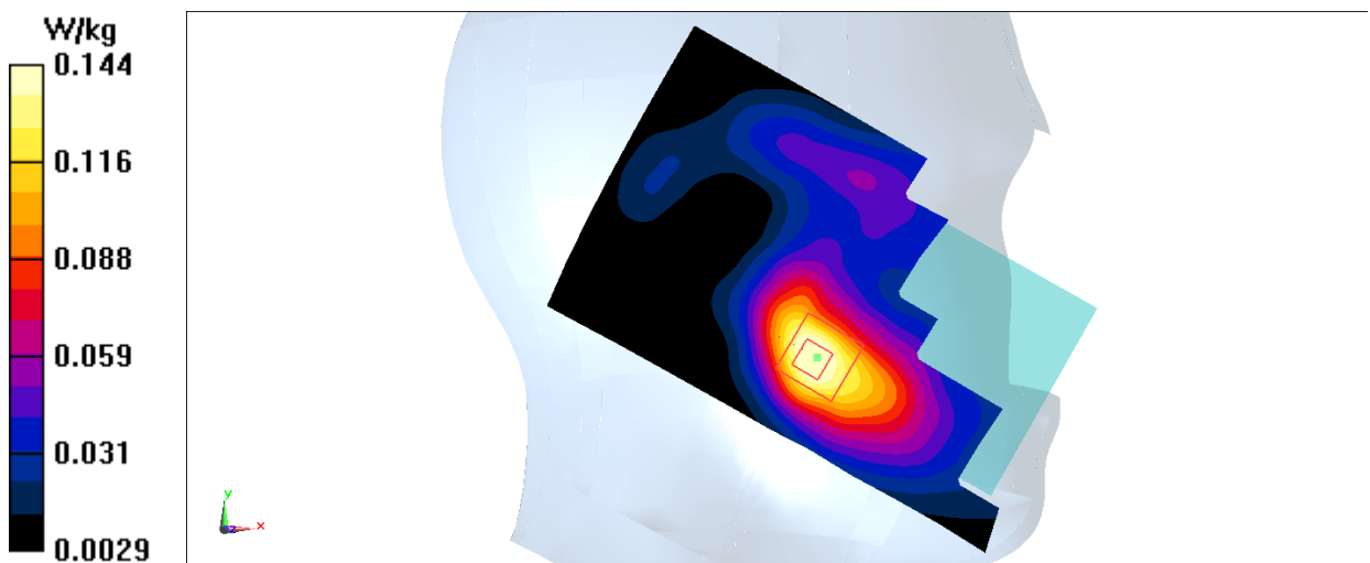
Fig.33 LTE Band66
