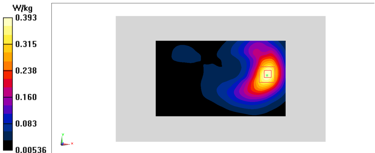
Fig.30 LTE Band30
