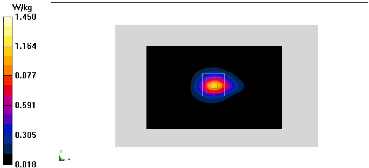
Fig.29 LTE Band30
