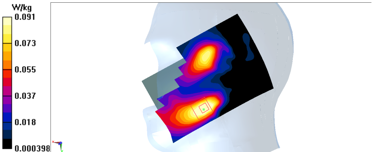
Fig.28 LTE Band30
