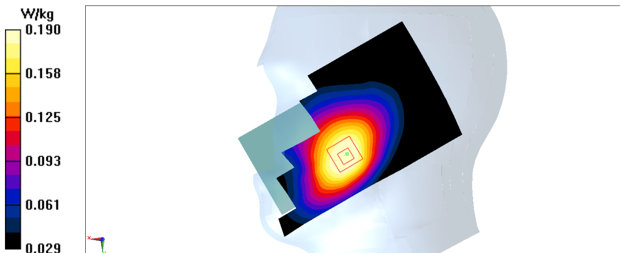
Fig.26 LTE Band14
