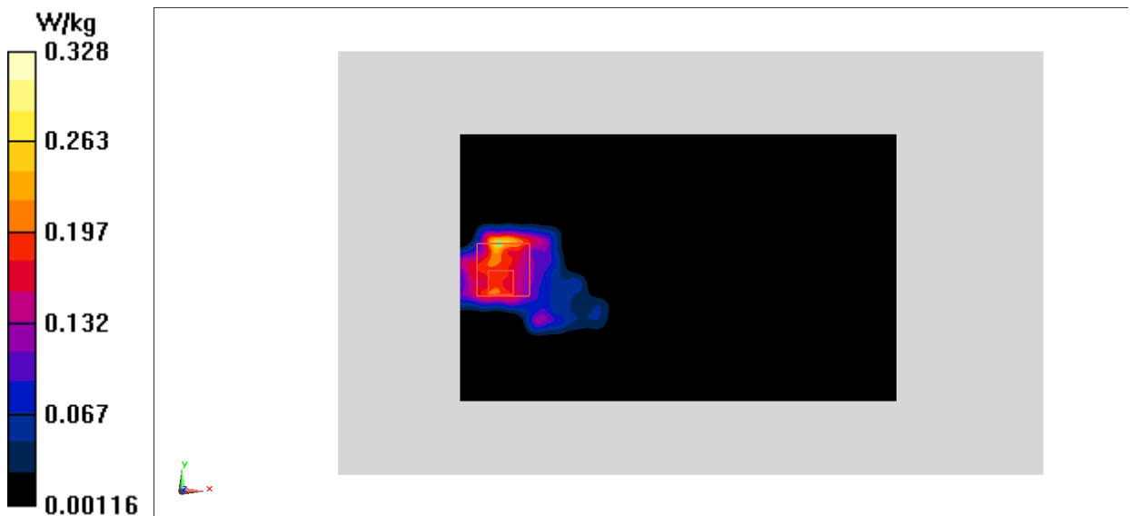
Fig.39 5GHz
