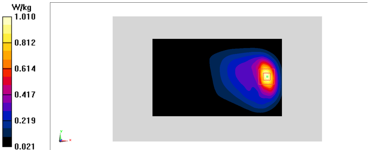
Fig.34 LTE Band66
