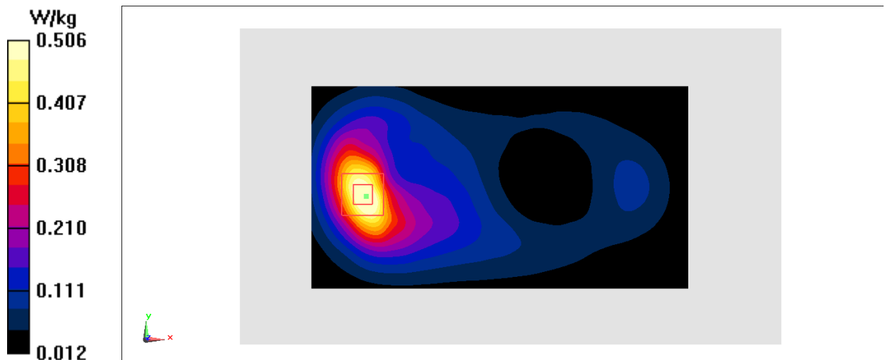
Fig.35 LTE Band66
