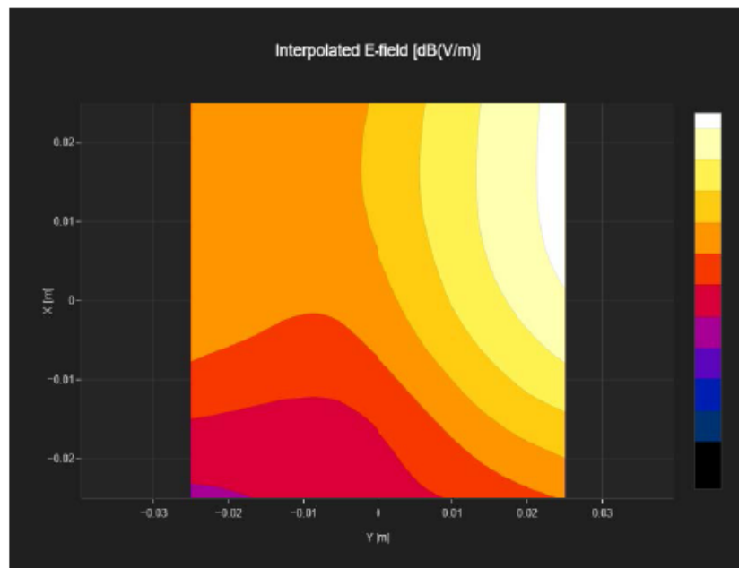
Fig F.4.2 HAC RF E-Field GSM1900
