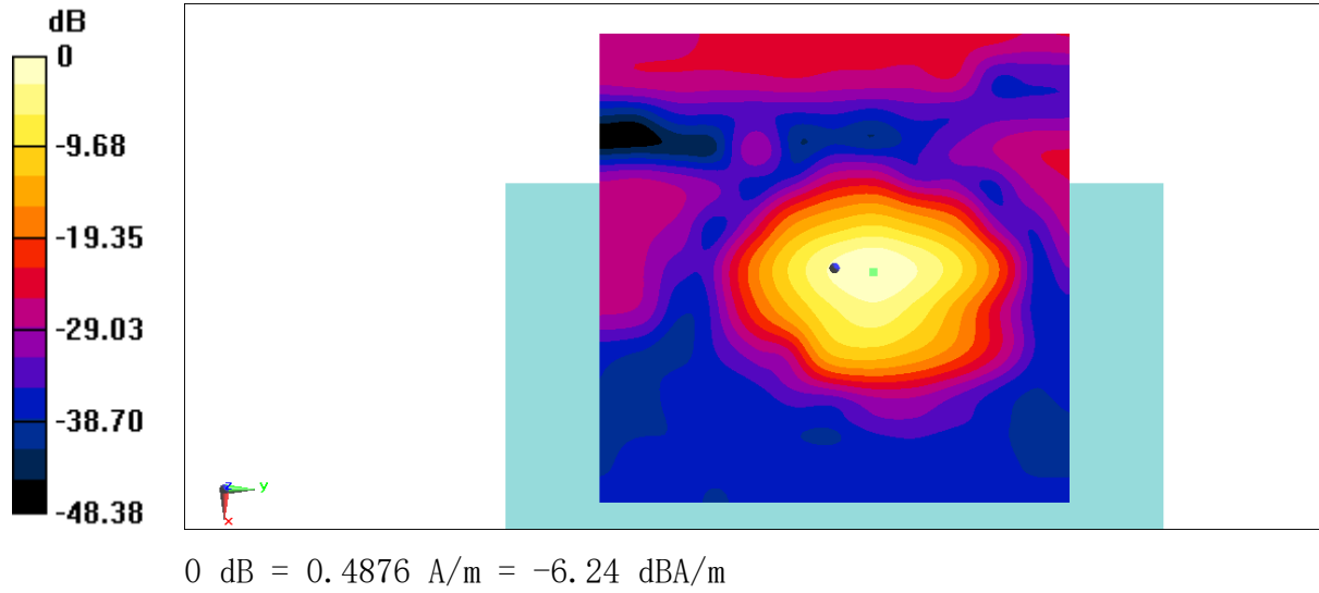
Fig B.12 T-Coil EDGE 1900
