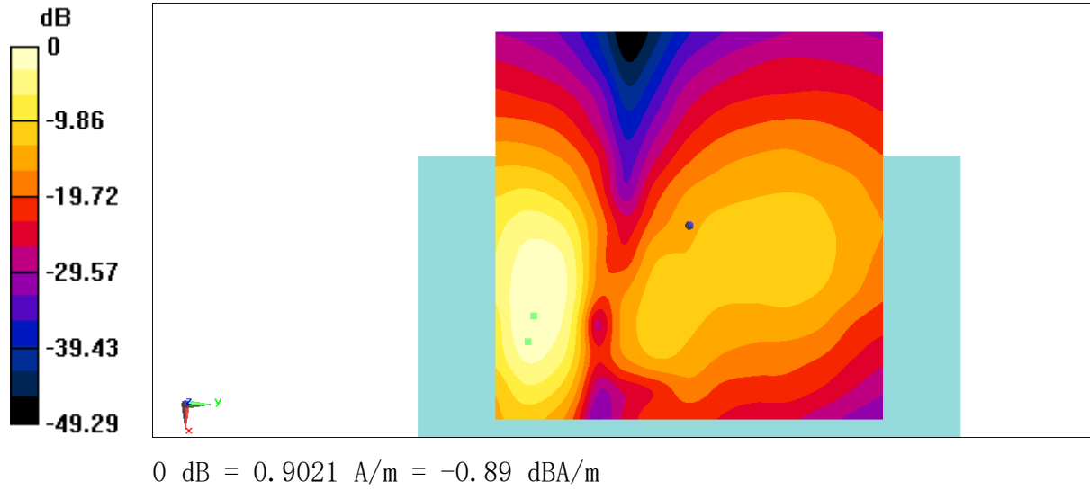
Fig B.7 T-Coil WiFi-2. 4G
