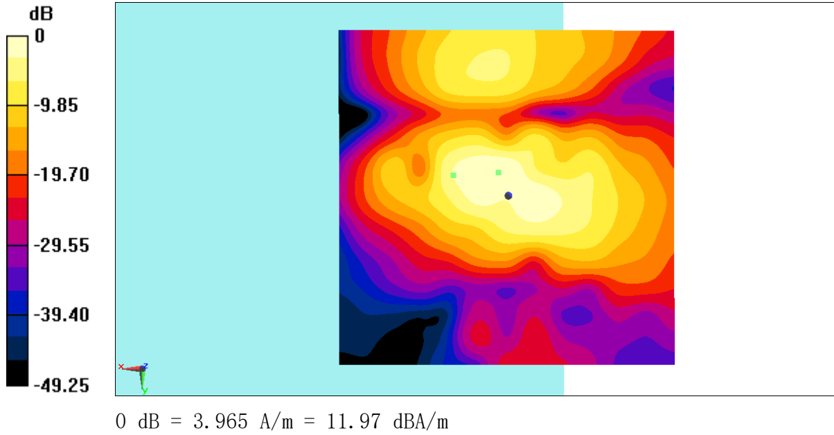
Fig F.3.13 T-Coil WiFi-2. 4G
