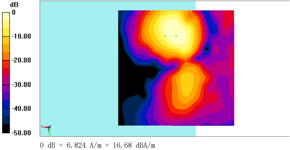
Fig F.3.12 T-Coil LTE B66 -0TT
