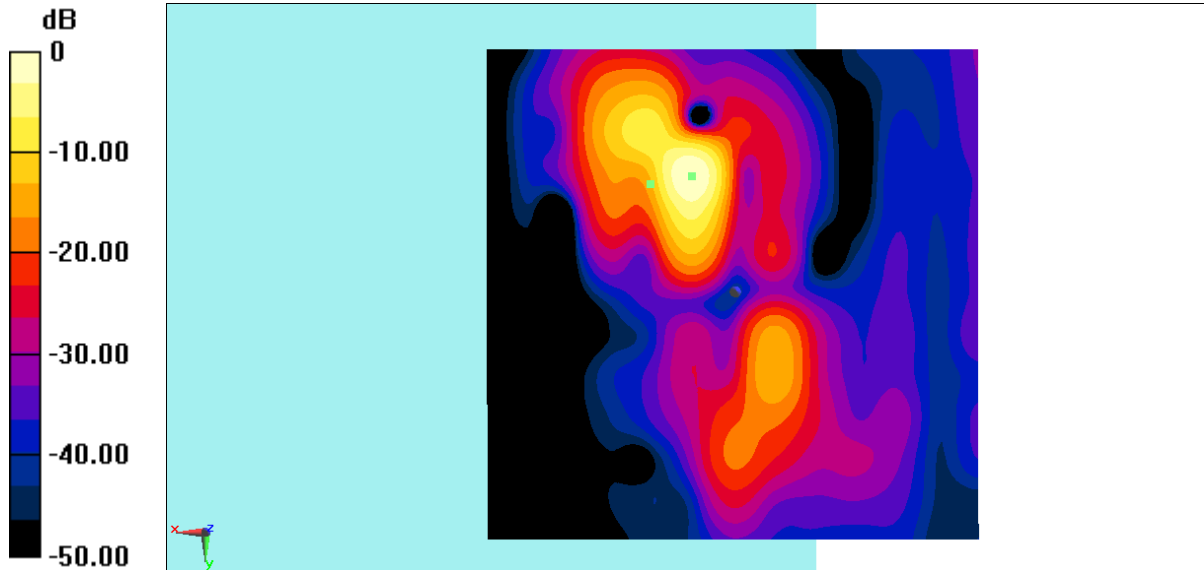
Fig F.3.14 T-Coil WiFi-2.4G
