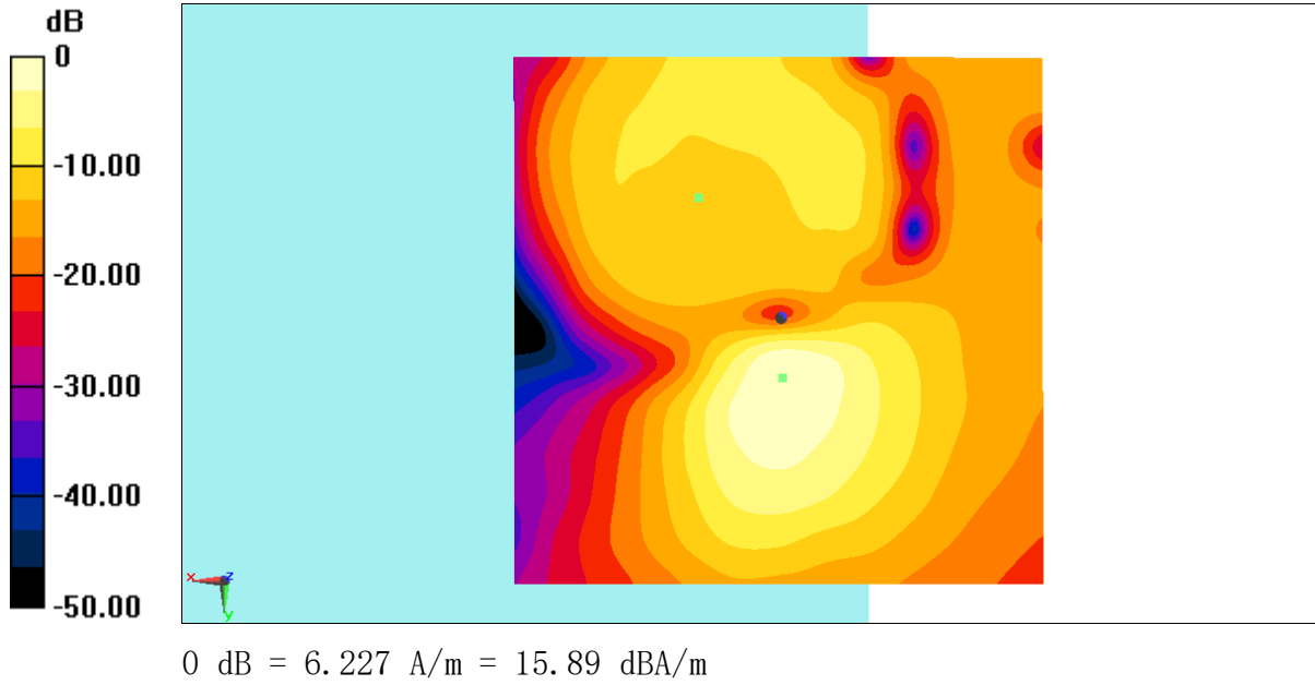
Fig E.3.4 T-Coil WCDMA 850
