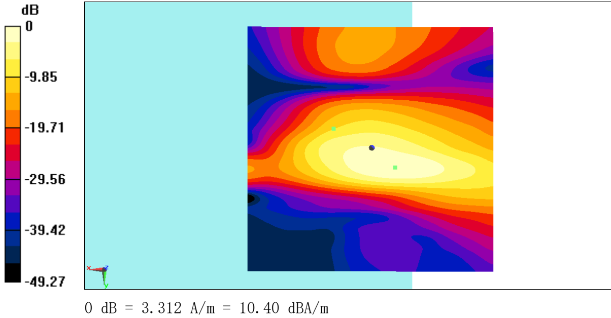
Fig F.3.1 T-Coil GSM 850
