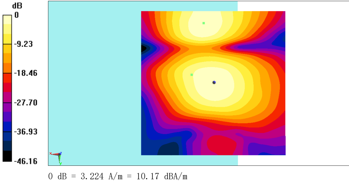
Fig F.3.9 T-Coil WCDMA 1900 -OTT
