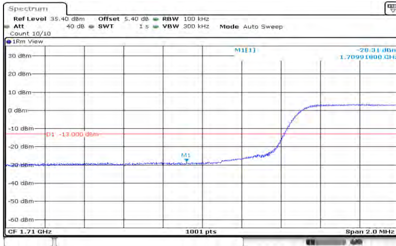
Band4-10MHz-QPSK-20000-50RB#0
