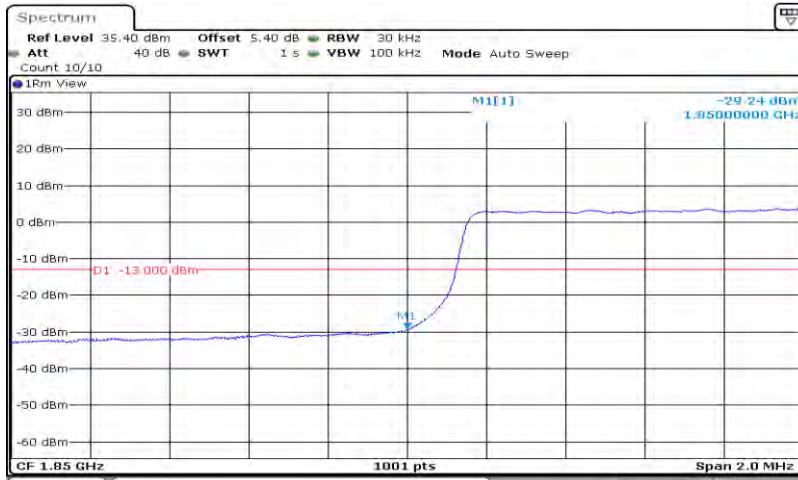
Band2-3MHz-QPSK-18615-15RB#0
