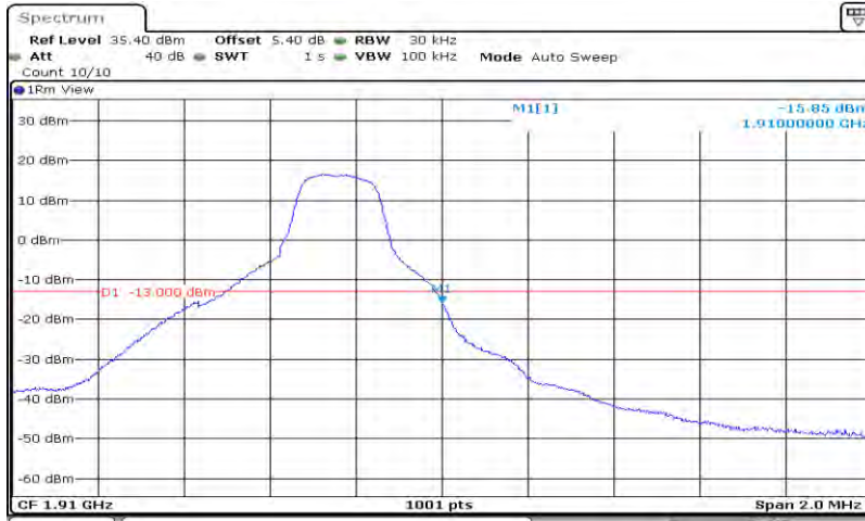
Band2-3MHz-QPSK-19185-15RB#0
