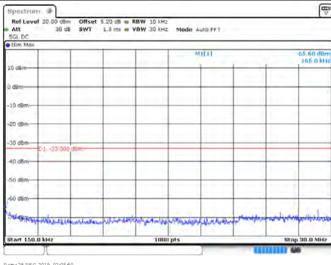
GSM1900_810
