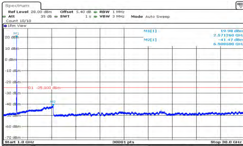
Band38-20MHz-16QAM-37850-1RB#0-Range2:1000~30000MHz
