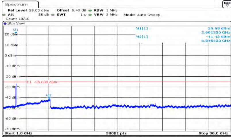
Band38-20MHz-QPSK-38150-1RB#0-Range2:1000~30000MHz
