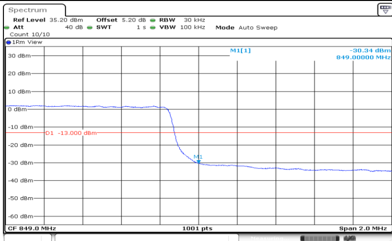
Band5-3MHz-QPSK-20635-15RB#0
