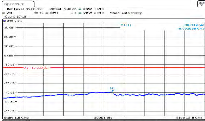
Band5-10MHz-QPSK-20525-1RB#0-Range2:1000~12000MHz
