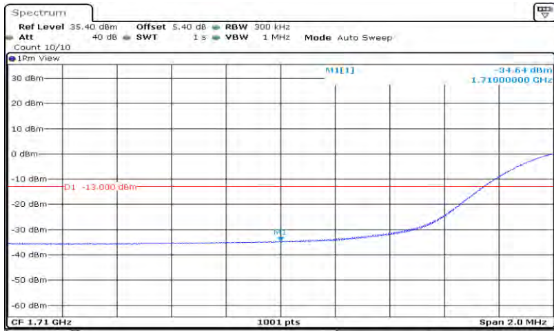
Band4-20MHz-QPSK-20050-100RB#0
