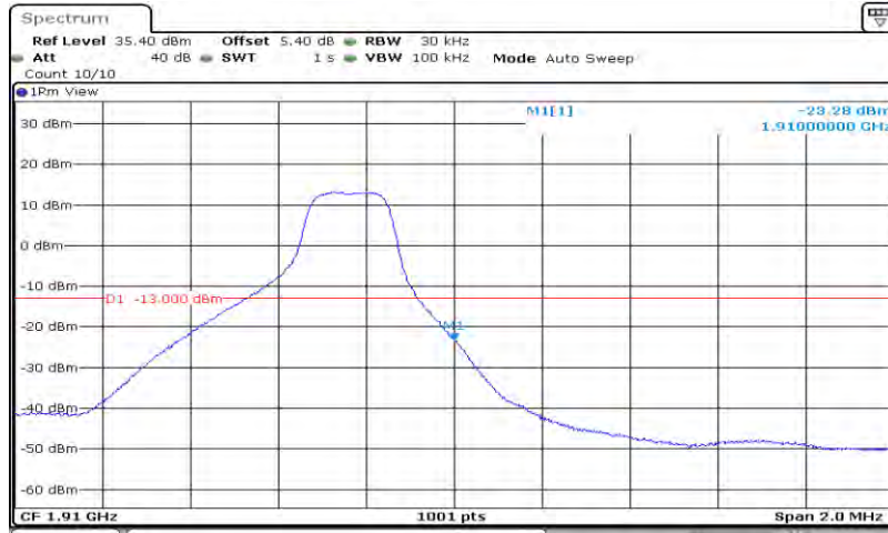
Band2-3MHz-QPSK-19185-15RB#0
