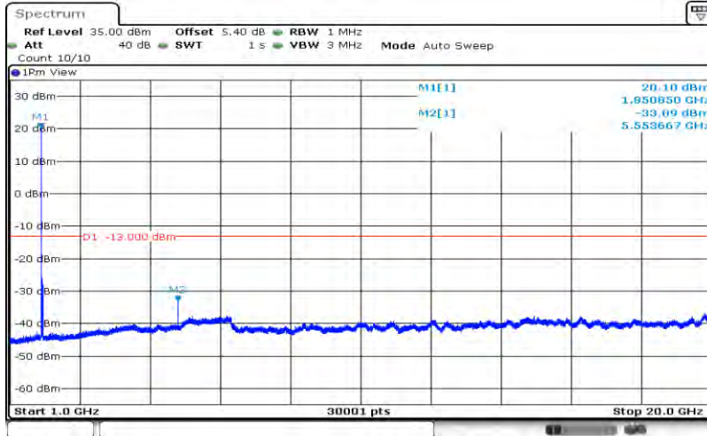
Band2-20MHz-16QAM-18700-1RB#0-Range2:1000~20000MHz
