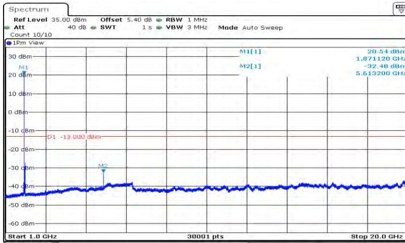
Band2-20MHz-16QAM-18900-1RB#0-Range2:1000~20000MHz
