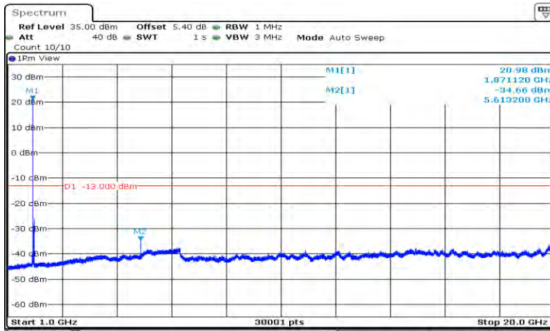
Band2-20MHz-QPSK-18900-1RB#0-Range2:1000~20000MHz
