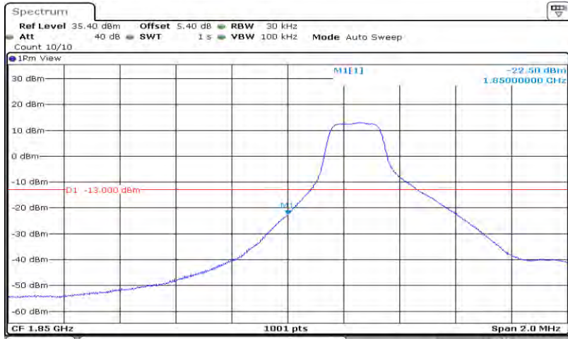
Band2-3MHz-16QAM-18615-15RB#0
