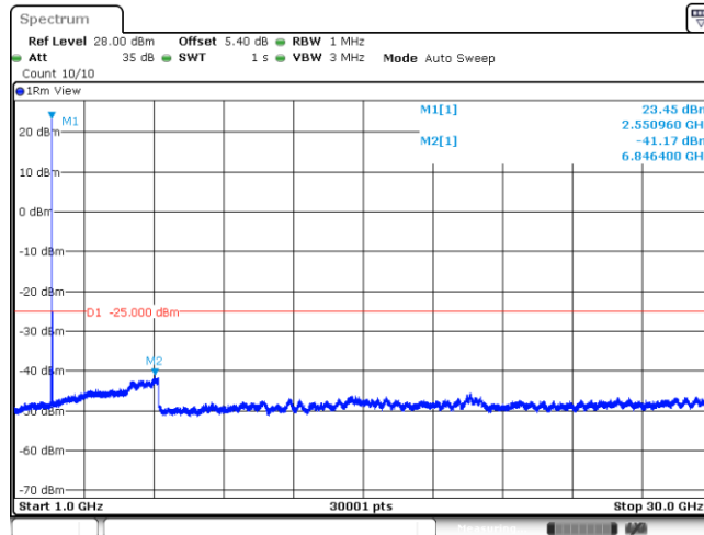
Band7_20MHz_QPSK_21350_1RB#0
