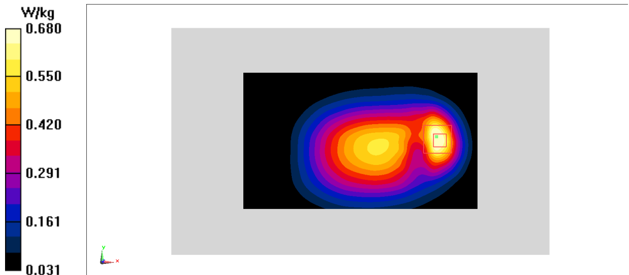
Fig.17 LTE Band5
