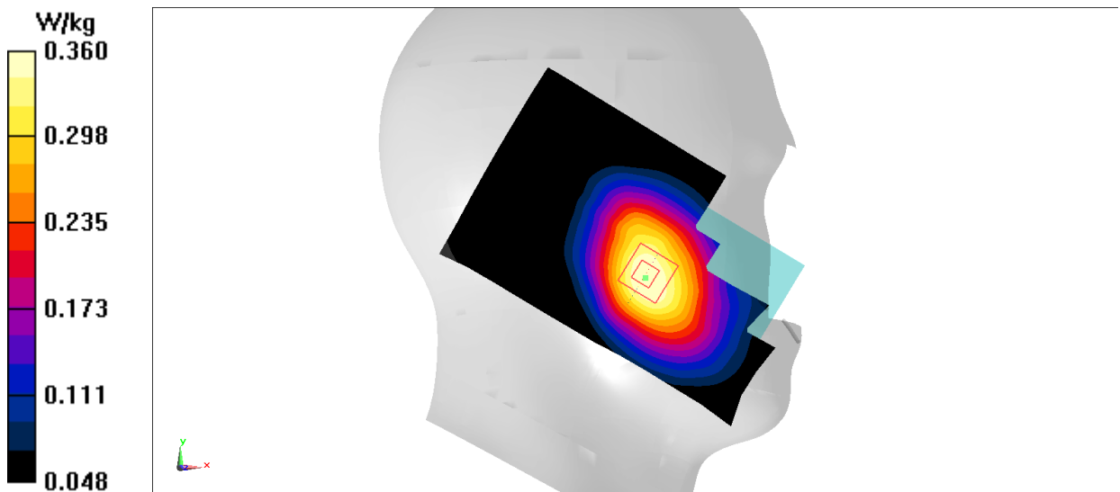
Fig.20 LTE Band13
