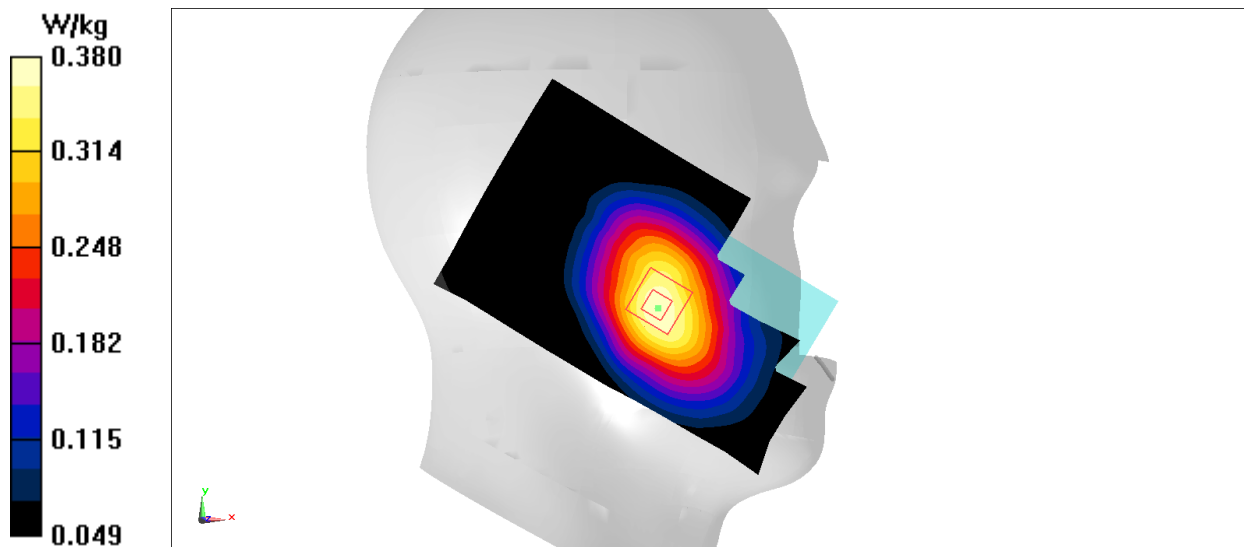
Fig.16 LTE Band5
