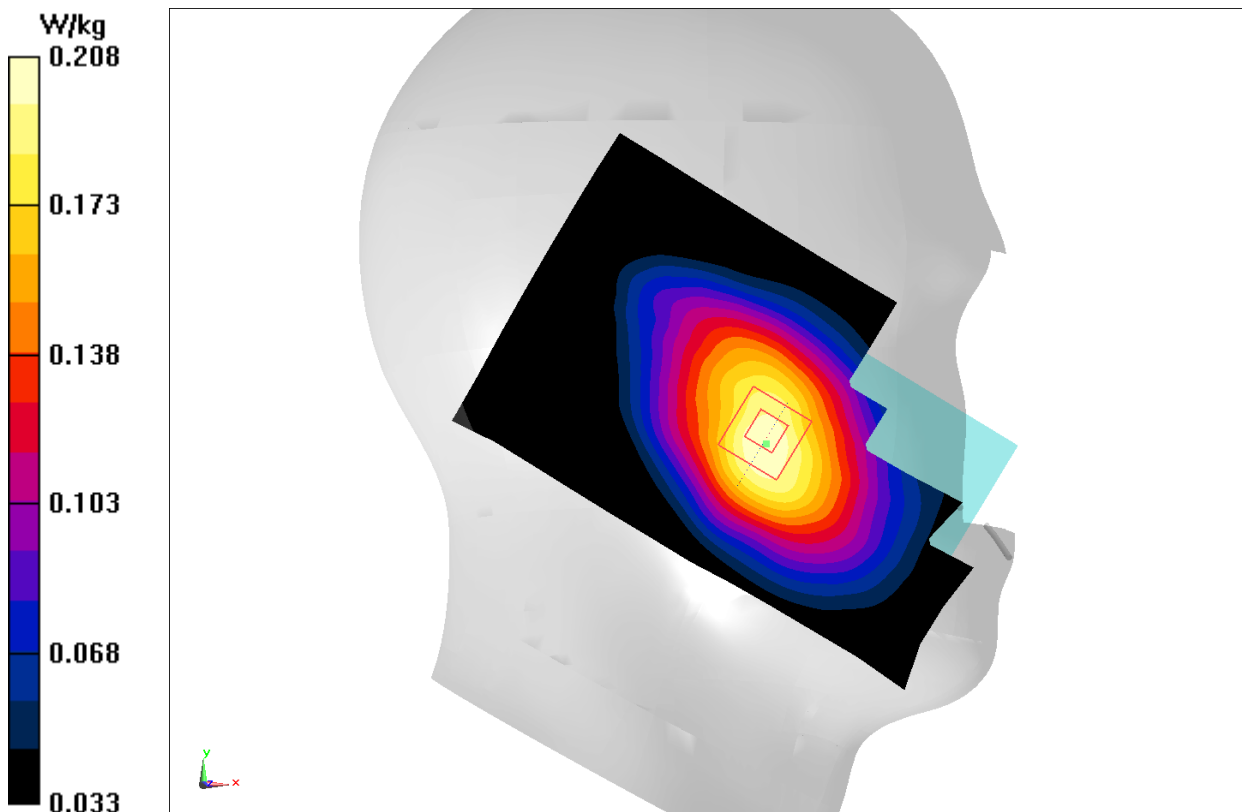
Fig.25 LTE Band71
