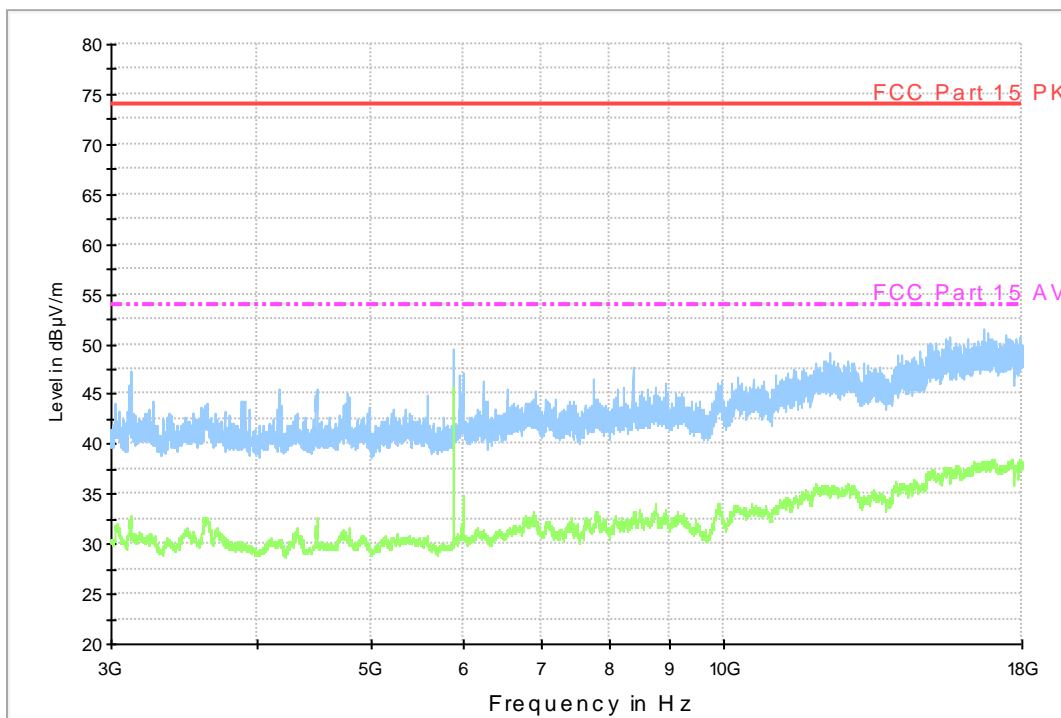
15b RE - 3GHz-18GHz
