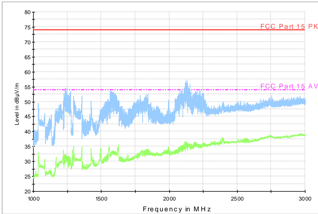
15B RE - 1GHz-3GHz
