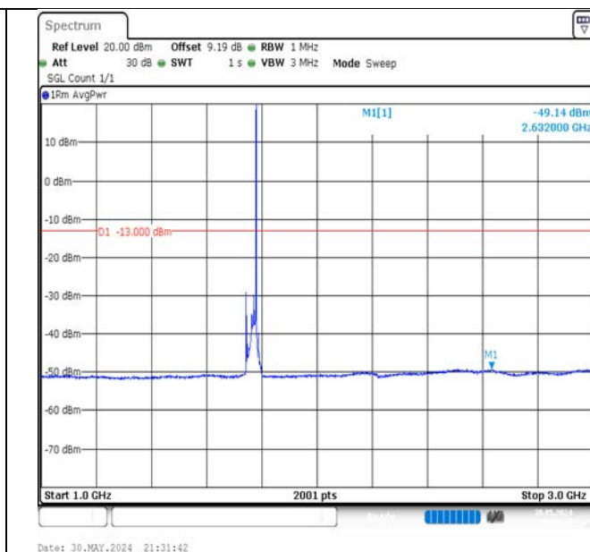
Band66-20MHz-QPSK-132572-1RB#99-1000~3000-PASS
