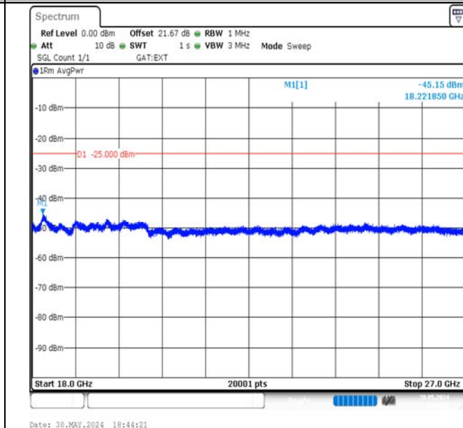
Band41-15MHz-16QAM-41515-1RB#74-18000~27000-PASS
