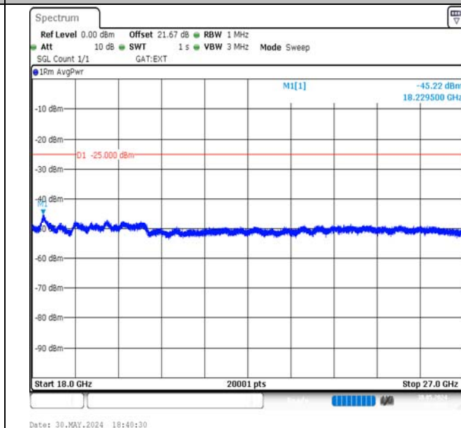
Band41-15MHz-16QAM-41515-1RB#0-18000~27000-PASS
