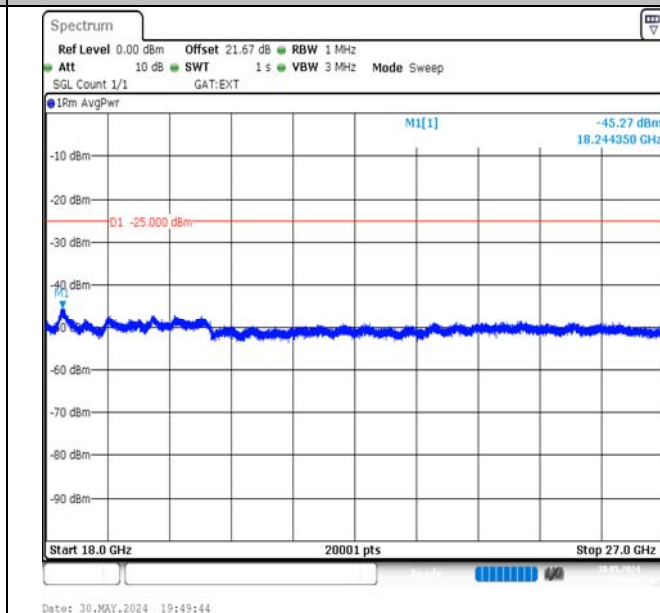
Band41-20MHz-16QAM-41490-1RB#0-18000~27000-PASS
