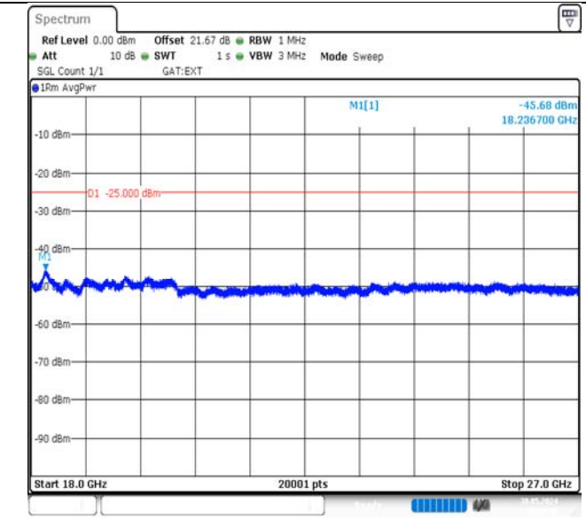
Band41-20MHz-QPSK-41490-1RB#0-18000~27000-PASS
