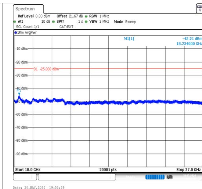
Band41-20MHz-QPSK-41490-1RB#99-18000~27000-PASS
