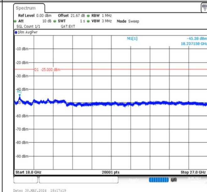
Band41-15MHz-16QAM-39725-1RB#0-18000~27000-PASS
