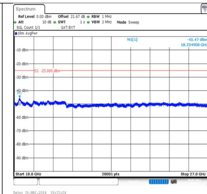
Band41-15MHz-QPSK-39725-1RB#0-18000~27000-PASS
