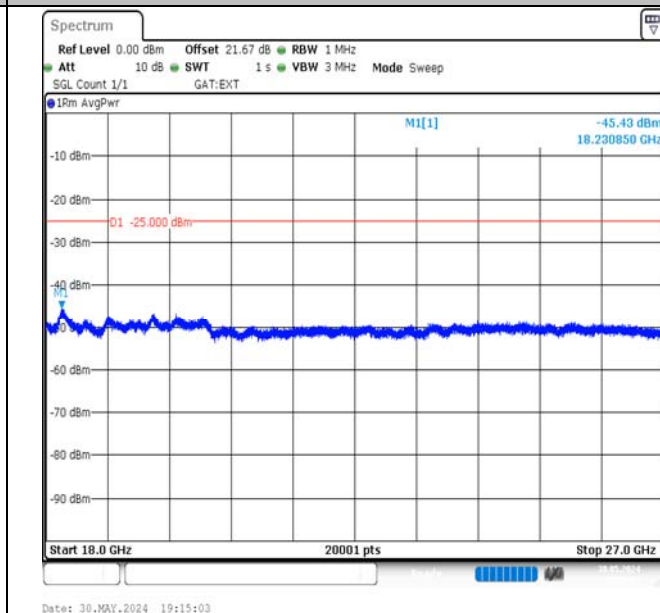
Band41-5MHz-16QAM-41565-1RB#0-18000~27000-PASS
