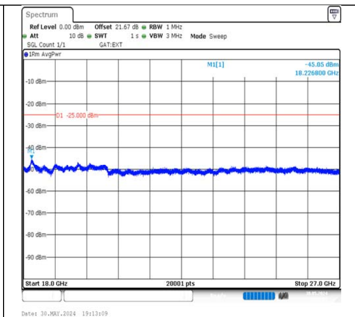
Band41-5MHz-QPSK-41565-1RB#0-18000~27000-PASS
