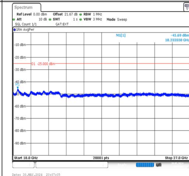
Band41-10MHz-QPSK-39700-50RB#0-18000~27000-PASS
