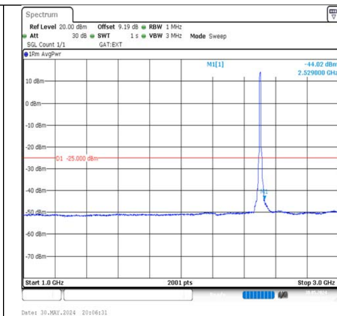
Band41-10MHz-QPSK-39700-50RB#0-1000~3000-PASS
