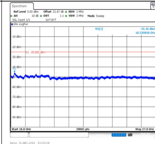
Band41-10MHz-QPSK-41540-50RB#0-18000~27000-PASS
