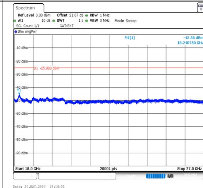
Band41-5MHz-16QAM-41565-1RB#24-18000~27000-PASS
