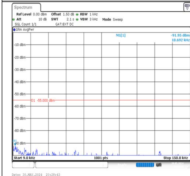
Band41-10MHz-QPSK-41540-50RB#0-0.009~0.15-PASS
