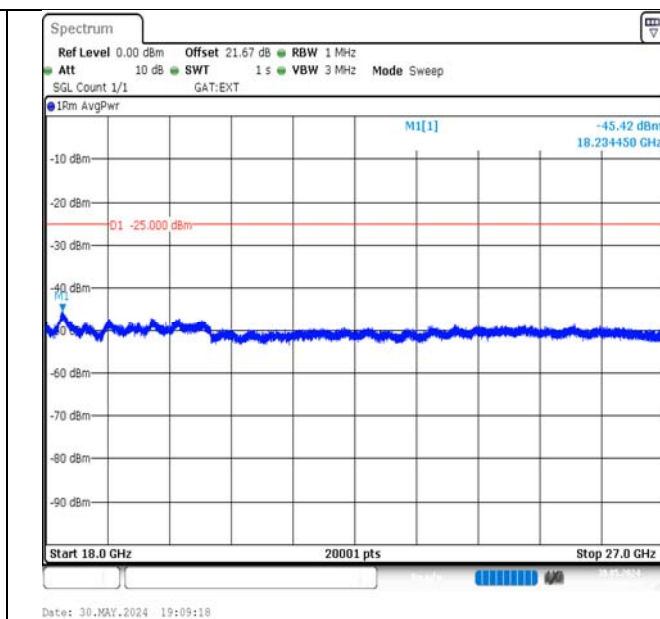
Band41-5MHz-QPSK-40620-25RB#0-18000~27000-PASS
