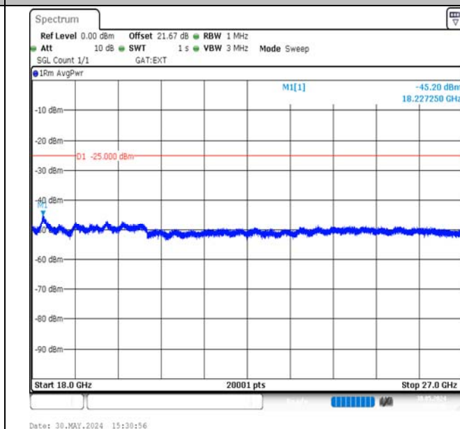
Band38-20MHz-QPSK-38000-1RB#99-18000~27000-PASS
