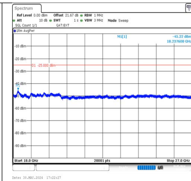
Band38-15MHz-QPSK-38175-1RB#0-18000~27000-PASS
