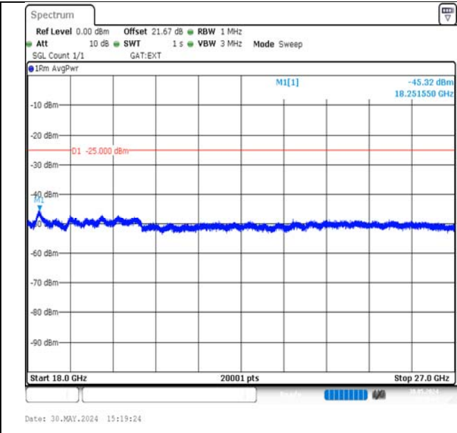
Band38-20MHz-QPSK-37850-1RB#99-18000~27000-PASS
