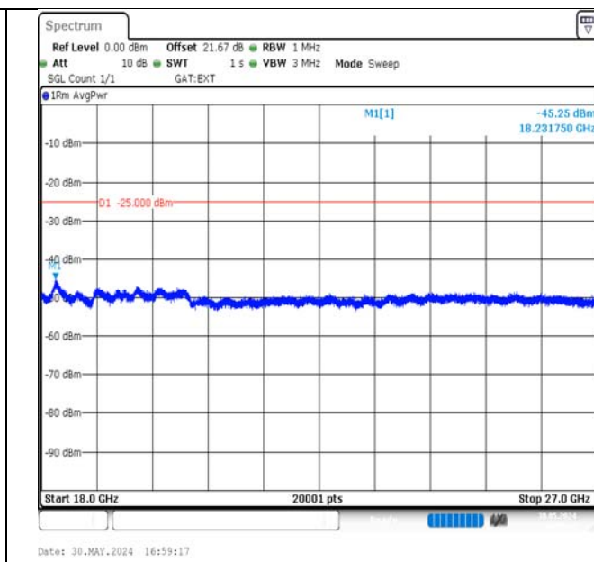
Band38-15MHz-QPSK-37825-1RB#0-18000~27000-PASS
