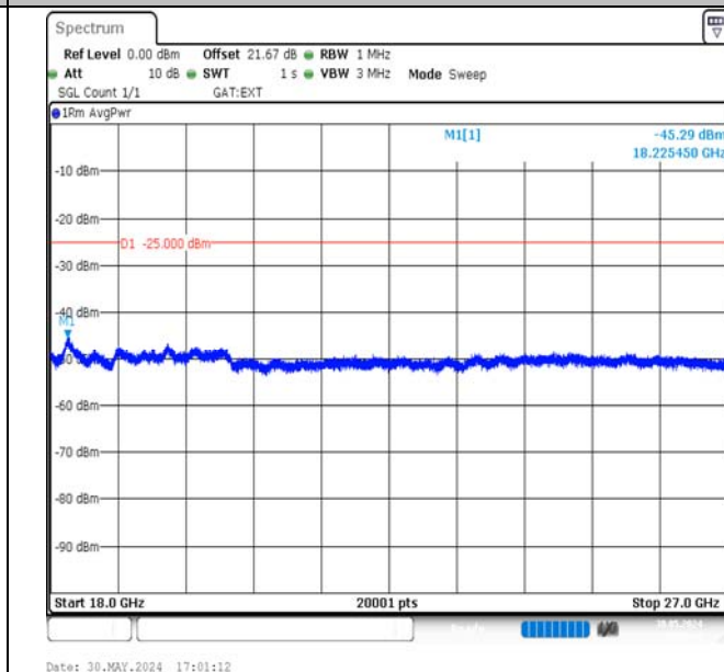
Band38-15MHz-16QAM-37825-1RB#0-18000~27000-PASS
