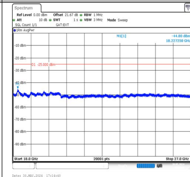
Band38-15MHz-QPSK-38000-1RB#74-18000~27000-PASS
