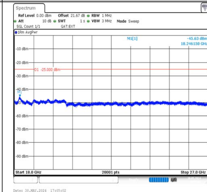
Band38-15MHz-16QAM-37825-1RB#74-18000~27000-PASS
