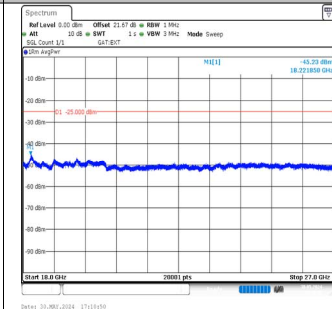
Band38-15MHz-QPSK-38000-1RB#0-18000~27000-PASS
