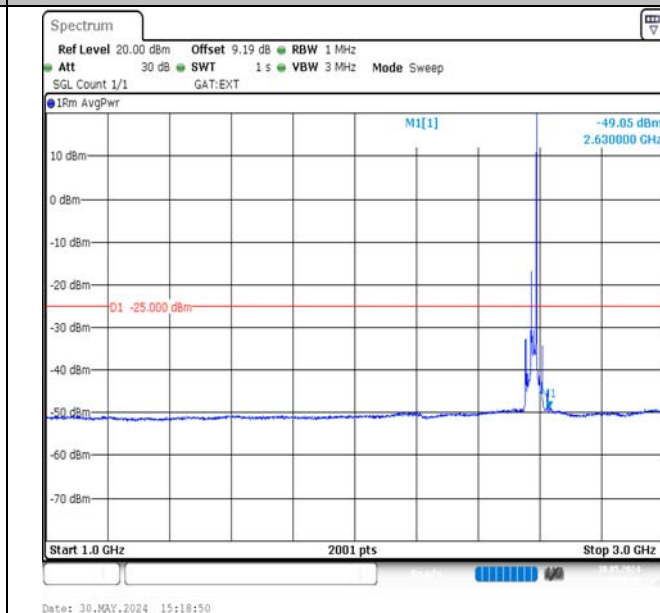
Band38-20MHz-QPSK-37850-1RB#99-1000~3000-PASS
