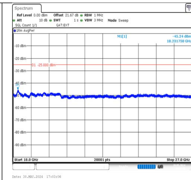
Band38-15MHz-QPSK-37825-1RB#74-18000~27000-PASS
