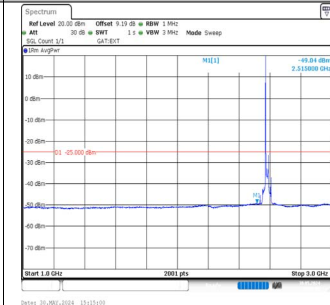
Band38-20MHz-QPSK-37850-1RB#0-1000~3000-PASS
