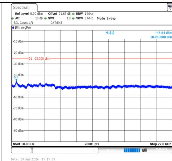
Band38-20MHz-QPSK-37850-1RB#0-18000~27000-PASS
