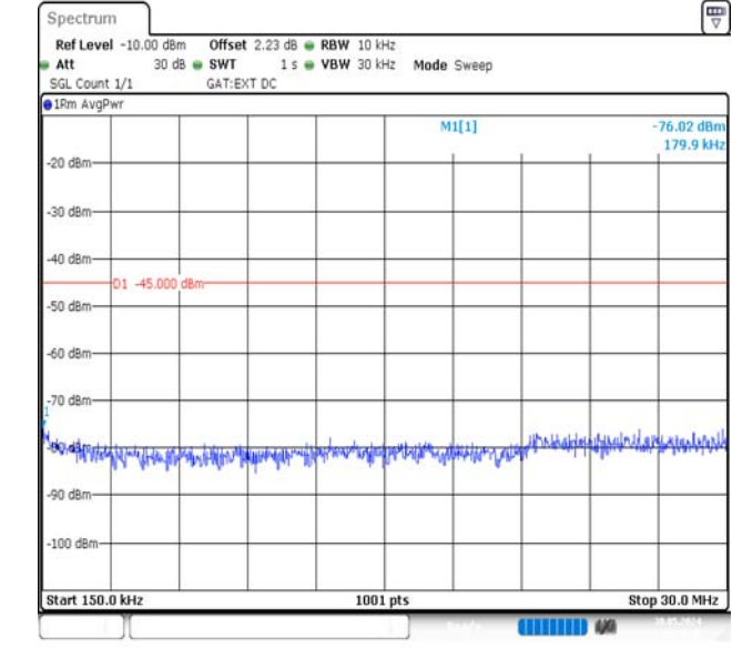
Band38-15MHz-16QAM-38000-1RB#0-18000~27000-PASS
