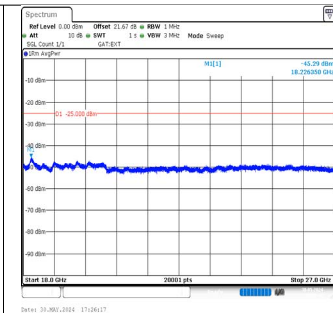
Band38-15MHz-QPSK-38175-1RB#74-18000~27000-PASS
