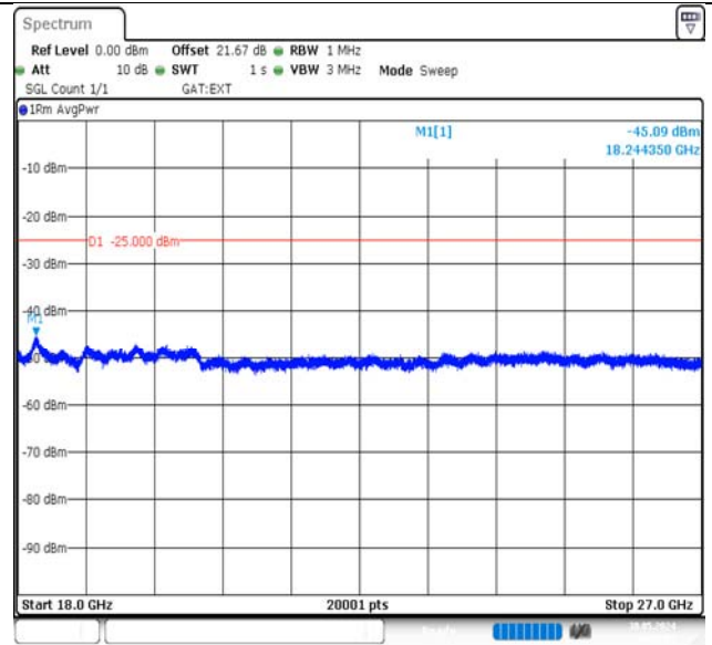
Band38-5MHz-QPSK-38000-25RB#0-18000~27000-PASS
