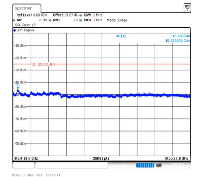
Band7-20MHz-QPSK-21350-1RB#99-18000~27000-PASS
