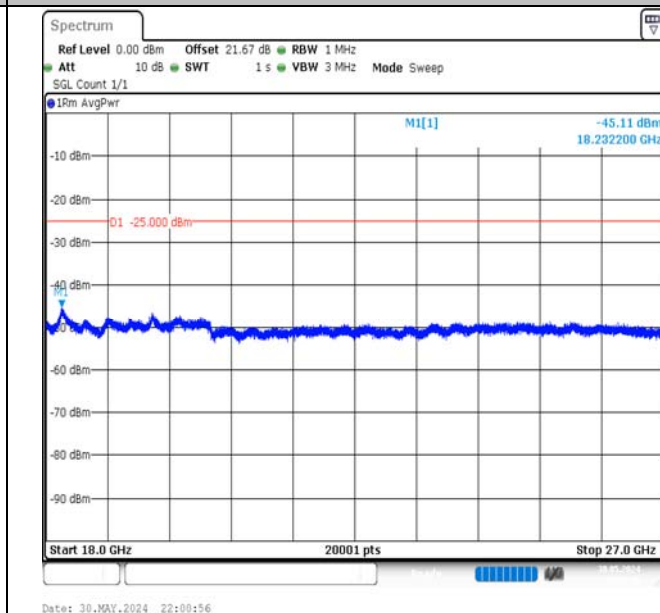
Band7-20MHz-QPSK-21100-1RB#99-18000~27000-PASS
