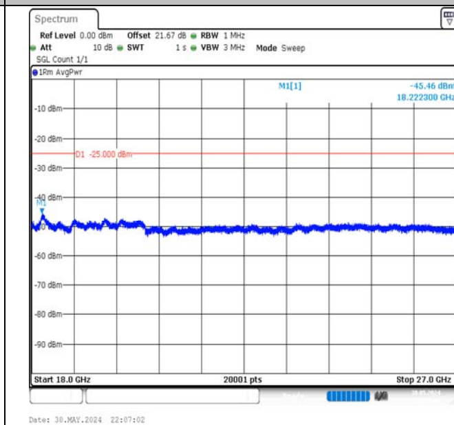
Band7-15MHz-16QAM-20825-1RB#74-18000~27000-PASS
