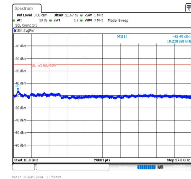
Band7-20MHz-QPSK-20850-1RB#99-18000~27000-PASS
