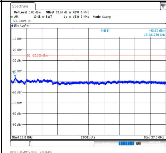
Band7-15MHz-16QAM-20825-1RB#0-18000~27000-PASS
