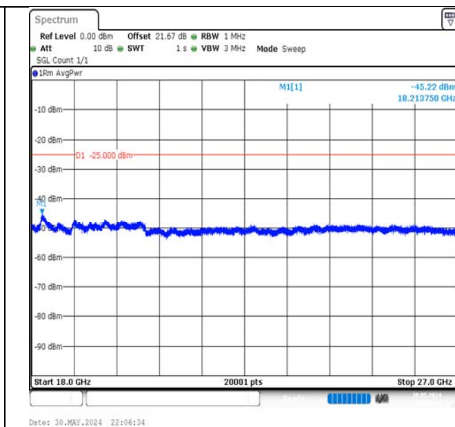
Band7-15MHz-QPSK-20825-1RB#74-18000~27000-PASS
