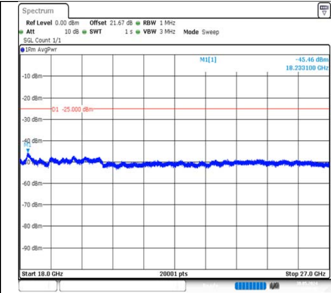
Band7-15MHz-QPSK-20825-1RB#0-18000~27000-PASS
