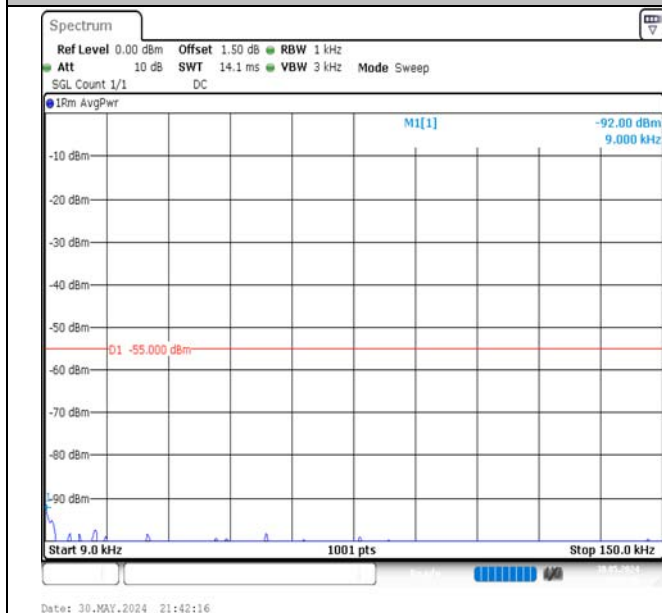
Band7-10MHz-QPSK-20800-50RB#0-0.009~0.15-PASS
