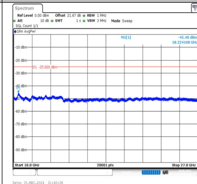
Band7-10MHz-QPSK-20800-50RB#0-18000~27000-PASS
