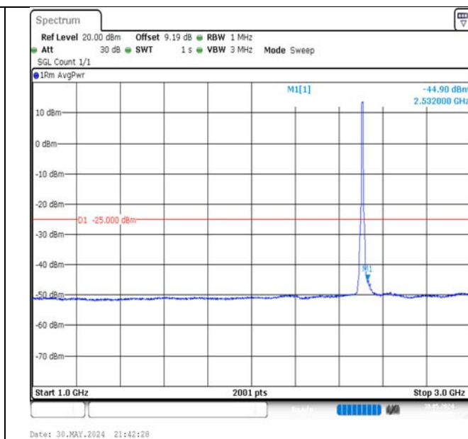
Band7-10MHz-QPSK-20800-50RB#0-1000~3000-PASS
