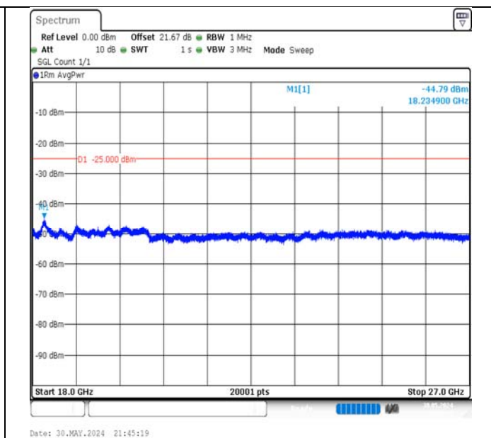
Band7-10MHz-QPSK-21100-50RB#0-18000~27000-PASS
