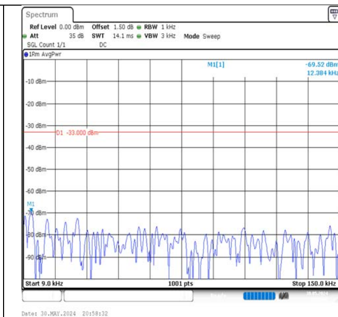
Band5-3MHz-QPSK-20635-15RB#0-0.009~0.15-PASS
