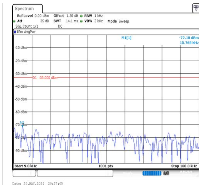
Band5-3MHz-QPSK-20635-1RB#0-0.009~0.15-PASS
