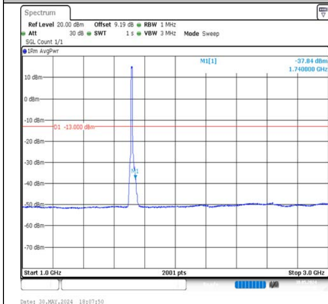
Band4-10MHz-QPSK-20000-50RB#0-1000~3000-PASS
