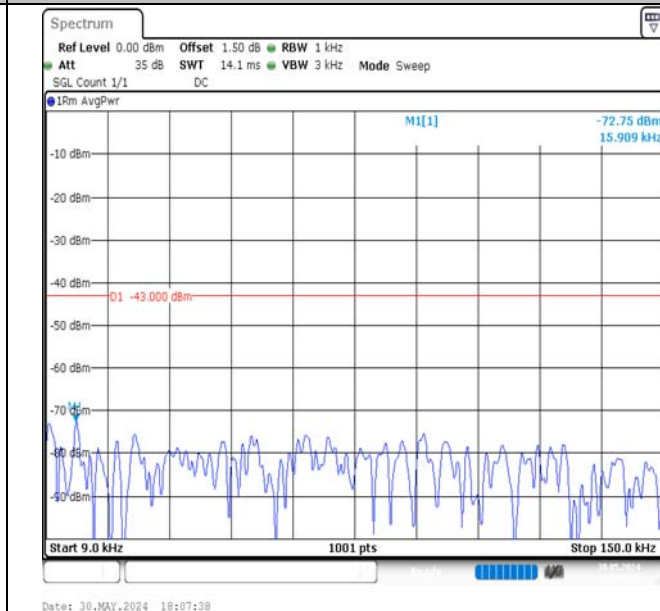
Band4-10MHz-QPSK-20000-50RB#0-0.009~0.15-PASS
